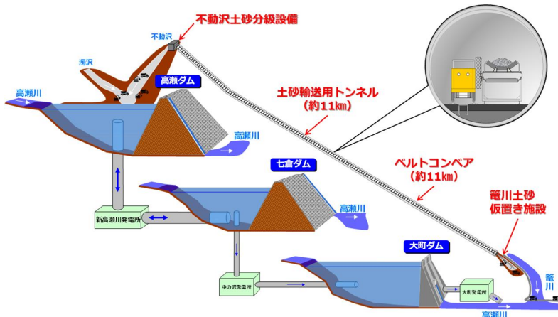
土砂輸送用トンネル・ベルトコンベア
