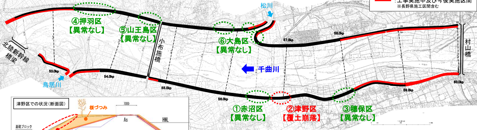
位置図(立ヶ花狭窄部～村山橋間)
