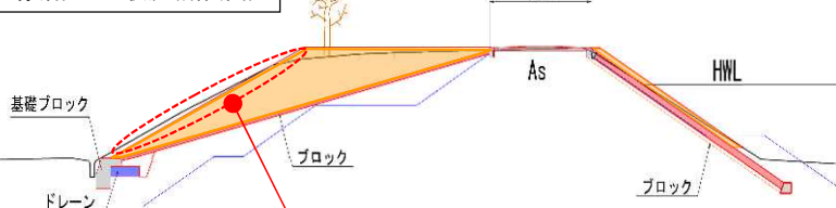
赤沼区での状況(断面図)
