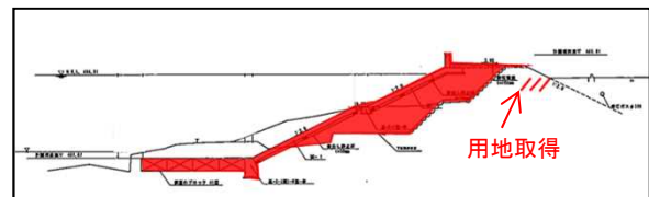
標準断面図
