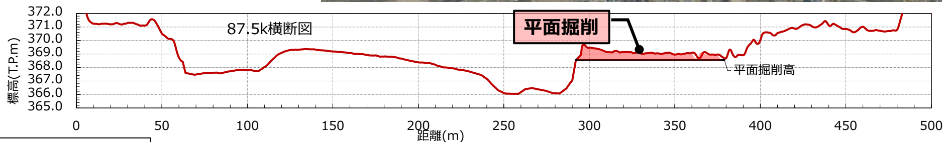
網掛地区掘削横断図
