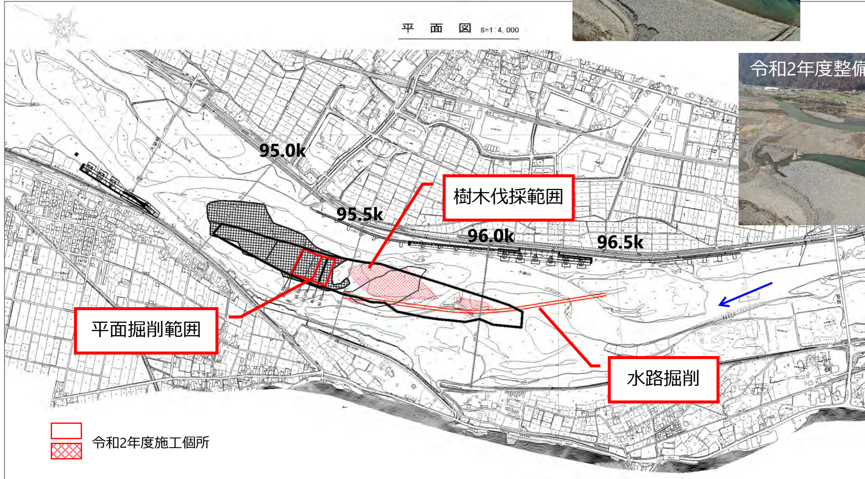
網掛地区整備図面（R2年度）
