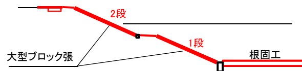
断面図
