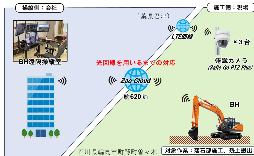
遠隔操縦概要図（（株）大林組提供）
