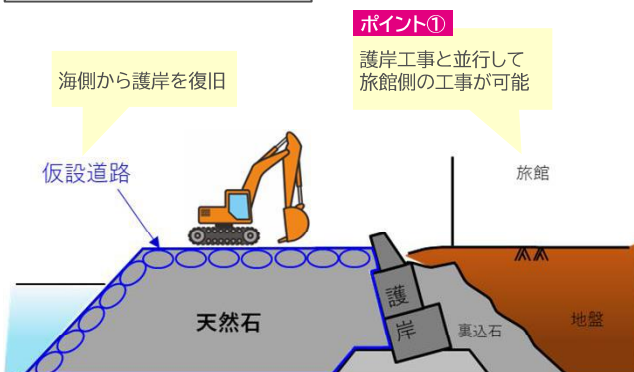
工事中(イメージ図)
