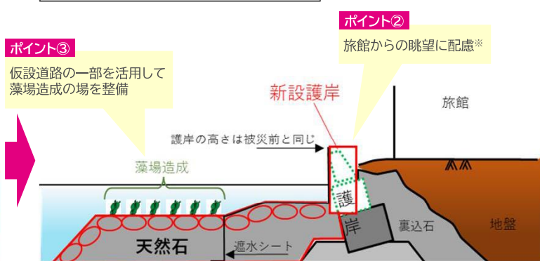
復旧等完了後(イメージ図)
