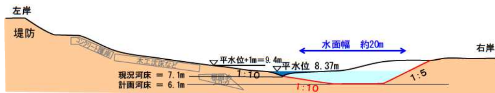
図 4.4-12 論瀬地区ワンドの計画断面図
