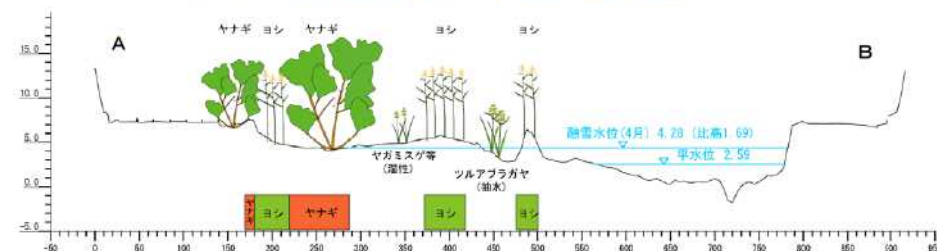
図 4. 6-2 ヤナギが再繁茂する地盤高と水位との関係整理例（中新田地区、平成 25 年度調査より）
