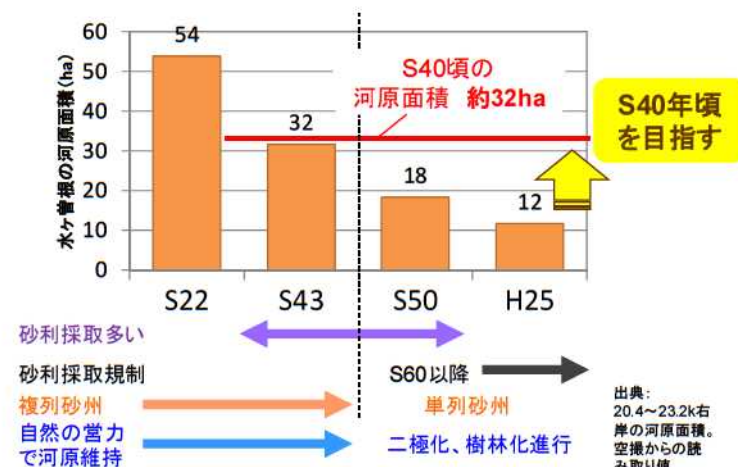
図 4.5-6 水ヶ曾根地区の河原面積の変遷
