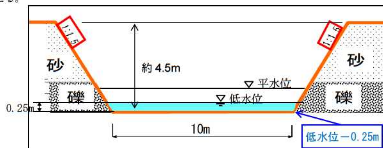
図 4.5-7 水ヶ曾根地区の断面形状（案）
