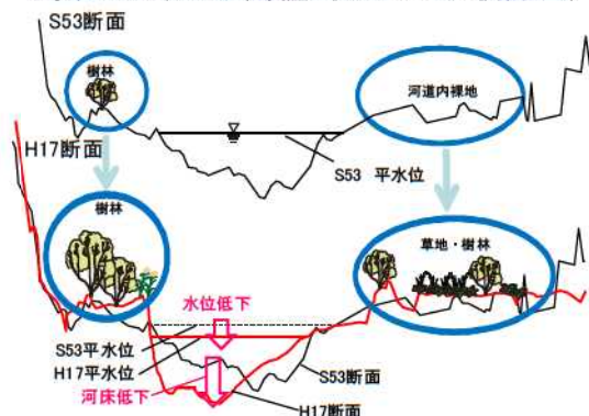
図 3.1-8 河床が低下し、水位が低下した 22.0k 断面（下流 2）
