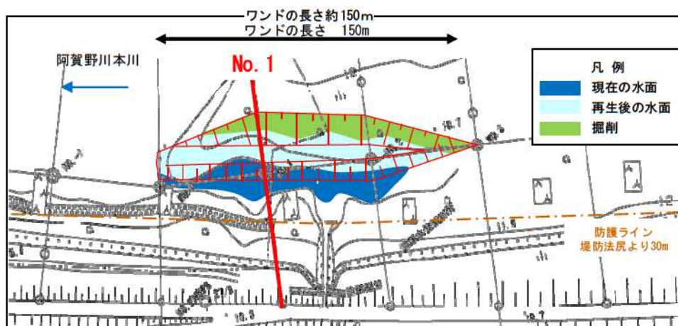
図 4.4-11 論瀬地区ワンドの計画平面図（イメージ）
