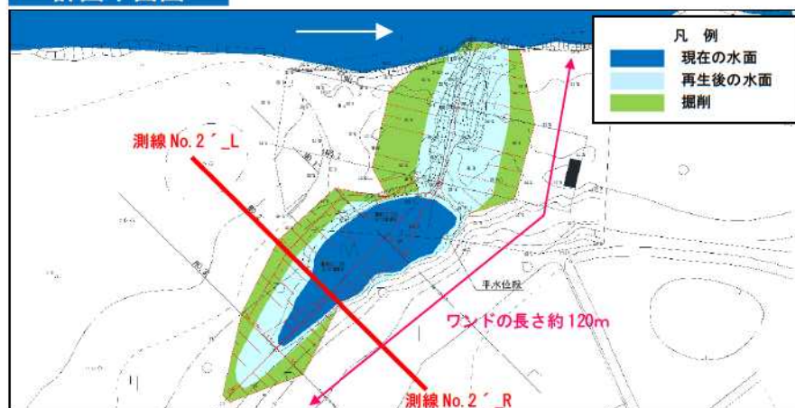
図 4.4-13 下里地区ワンドの計画平面図
