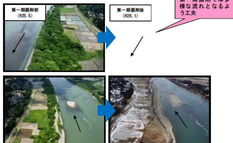
図 4.5-9 笹堀地区の第一期掘削の事例
