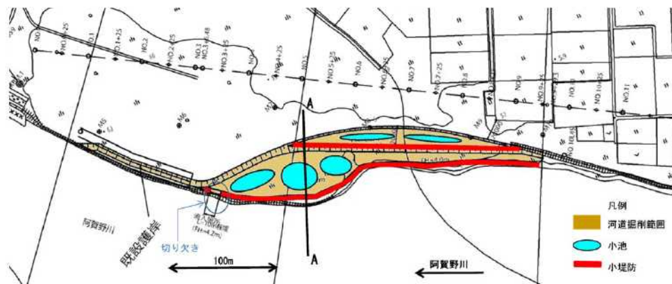
図 4.5-13 平面図
