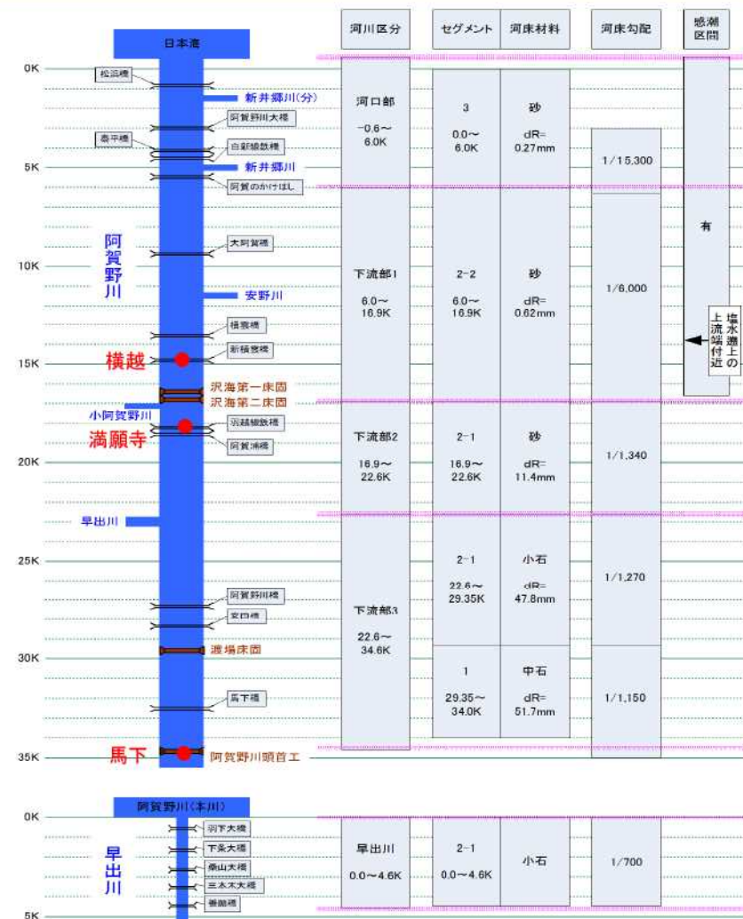
図 2.1-3 河道特性
