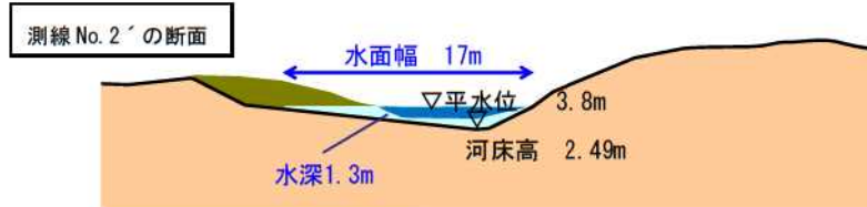
図 4.4-14 下里地区ワンドの計画断面図
