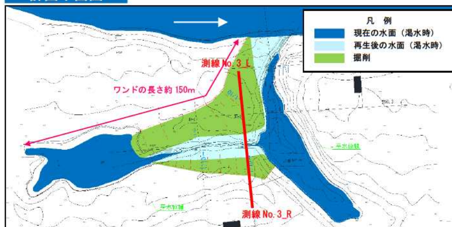
図 4.4-15 水ヶ曽根地区ワンドの計画平面図
