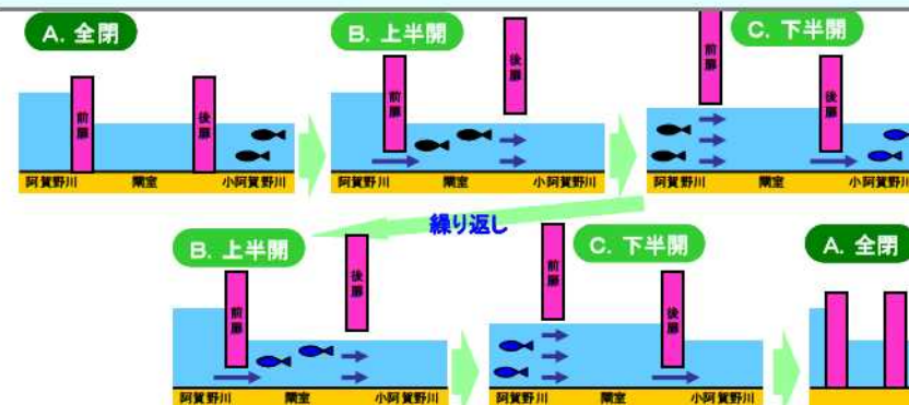
図 4.9-3 満願寺開門自動化によるアユの遡上を支援する操作のイメージ
