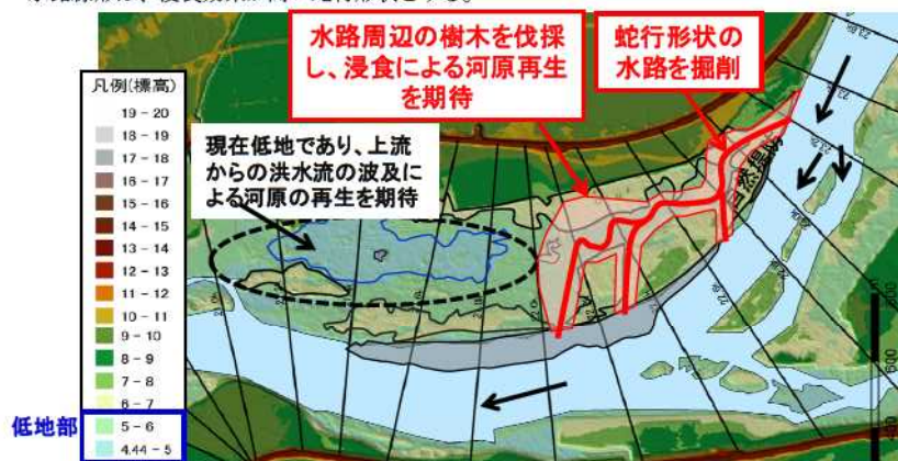
図 4.5-7 水ヶ曾根地区の平面形状（案）
