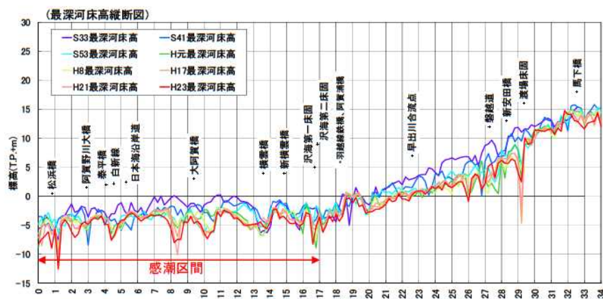
図 2.1-2 河川縦断面図
