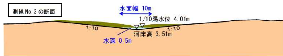
図 4.4-16 水ヶ曽根地区ワンドの計画断面図
