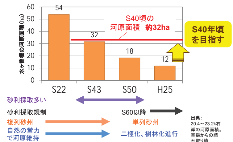
図 4.5-6 水ヶ曾根地区の河原面積の変遷
