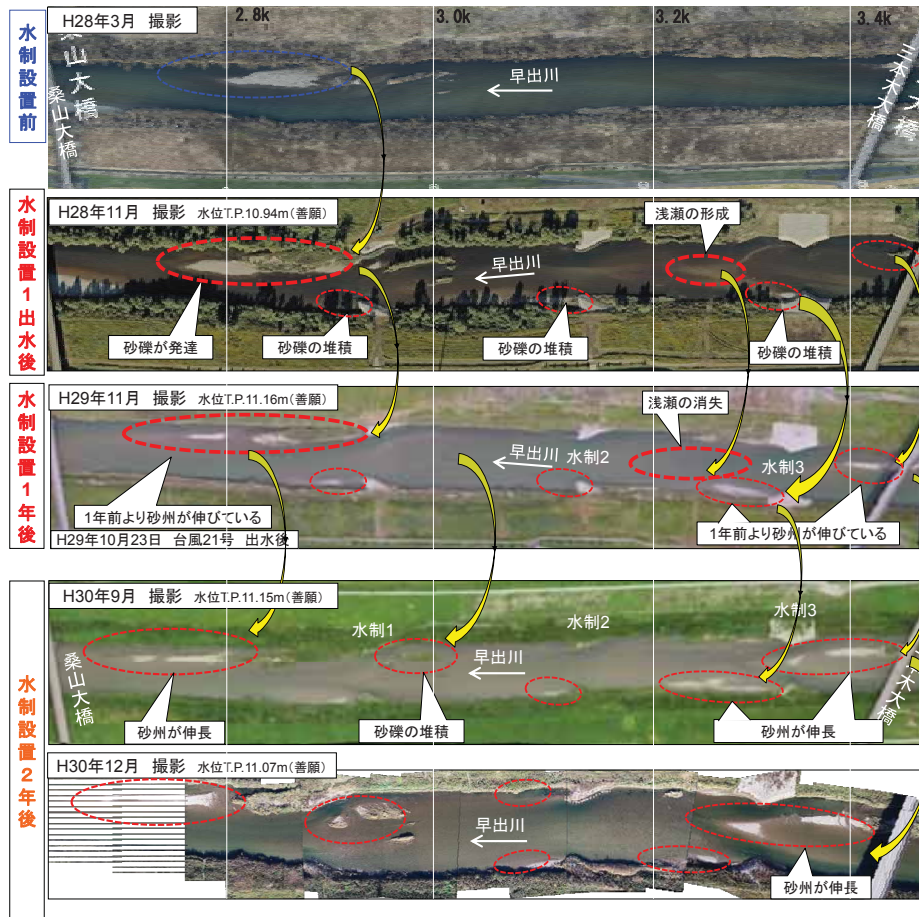
図 4.7-2 水制の設置による多様な流れの再生状況
