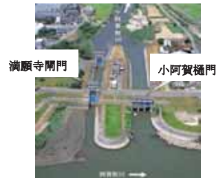
写真 3.2-10 小阿賀樋門及び満願寺開門
