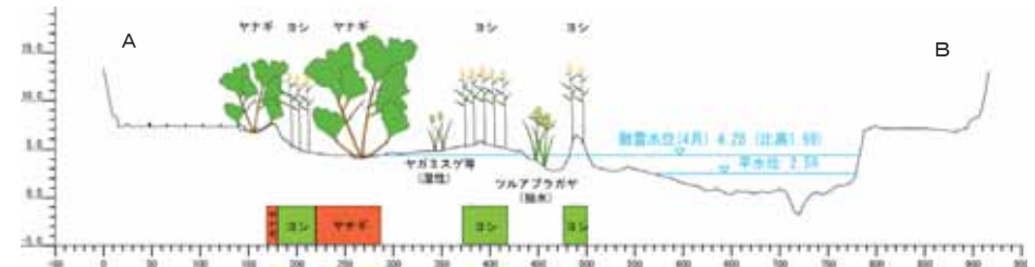
図 4.6-2 ヤナギが再繁茂する地盤高と水位との関係整理例（中新田地区、平成 25 年度調査より）
