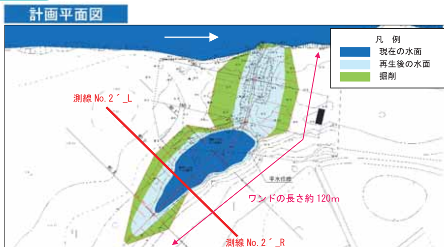
図 4.4-13 下里地区ワンドの計画平面図
