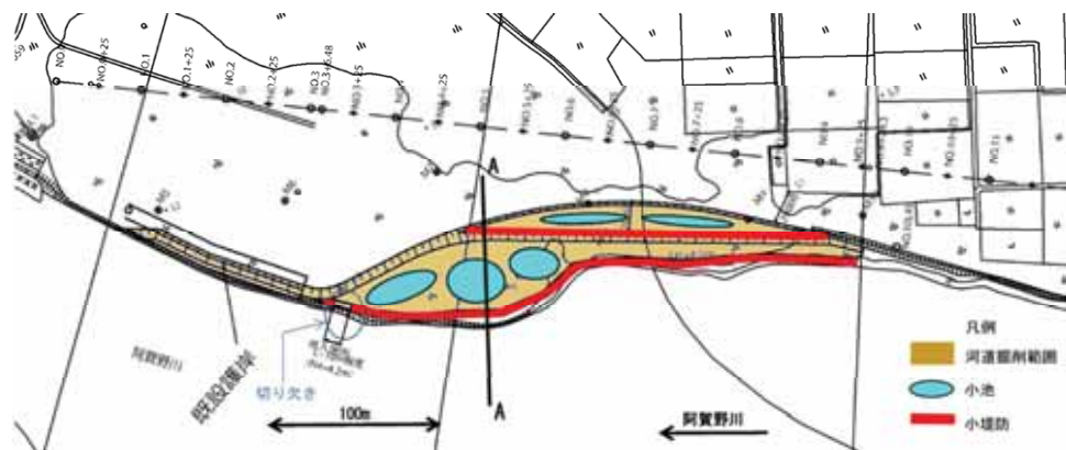
図 4.5-13 平面図
