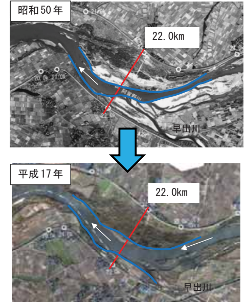
図 3.1-9 早出川合流点付近の河川形態
