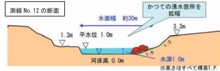
図 4.4-7 焼山地区ワンドの計画断面図
