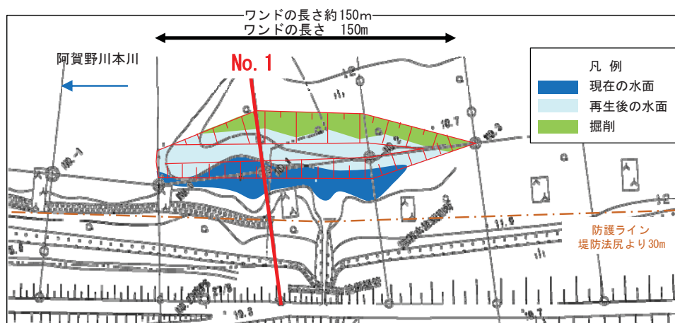
図 4.4-11 論瀨地区ワンドの計画平面図（イメージ）
