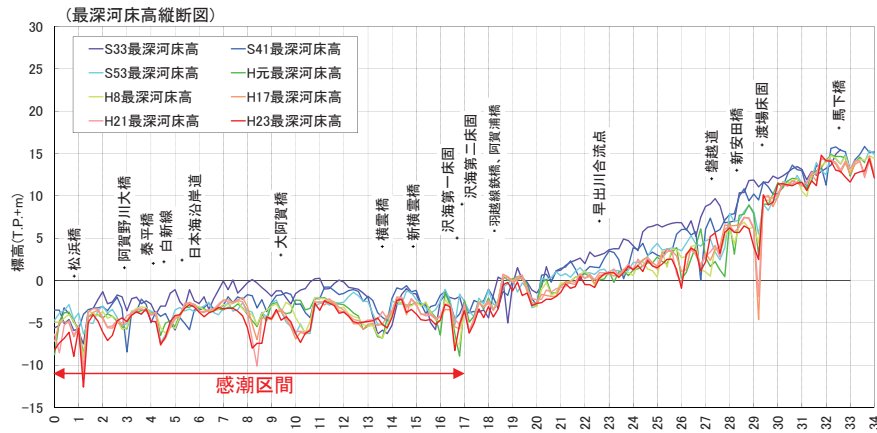
図 2.1-2 河川縦断面
