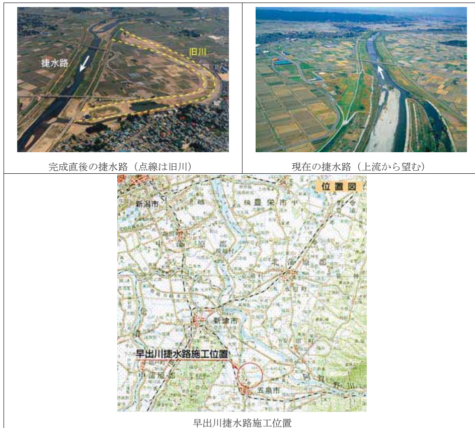
図 1.6-2 早出川捷水路の改修状況
