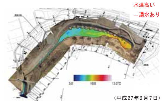
図 4.4-8 整備後の湧水位置の確認
