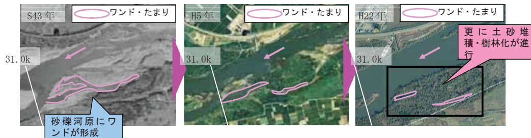
写真 4.4-3 高山地区の変遷
