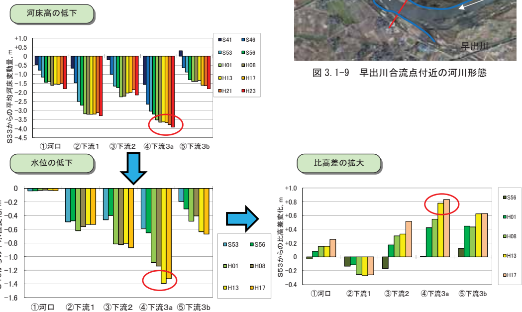
図 3.1-10 河床高・水位・比高差の変化
