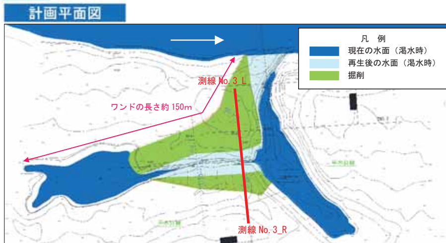
図 4.4-15 水ヶ曽根地区ワンドの計画平面図
