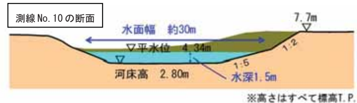
図 4.4-10 高山地区ワンドの計画断面図
