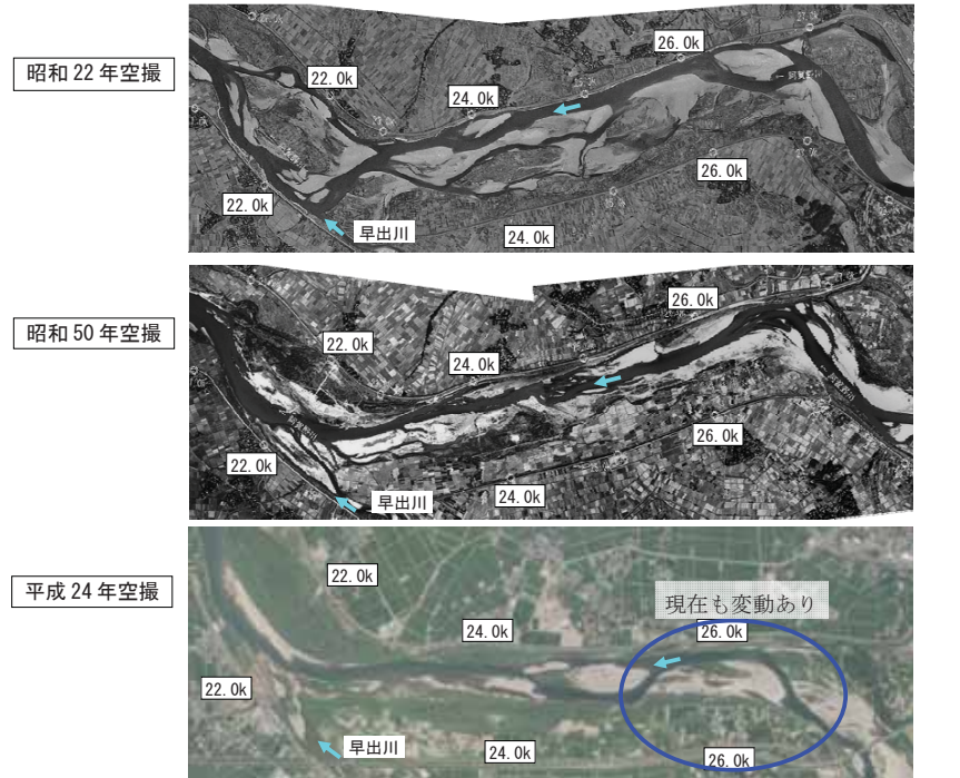
図 3.1-6 滞筋の変遷
