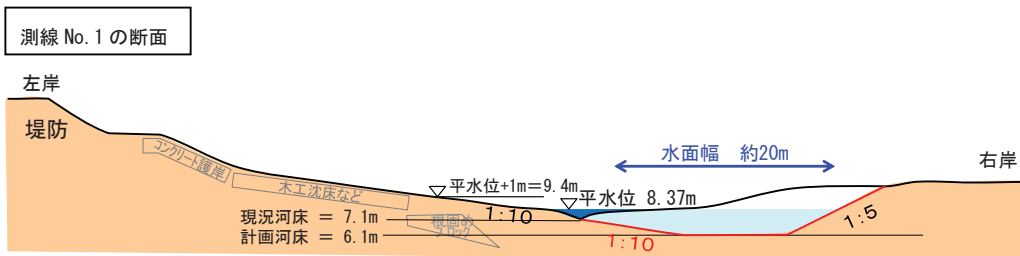
図 4.4-12 論瀨地区ワンドの計画断面図
