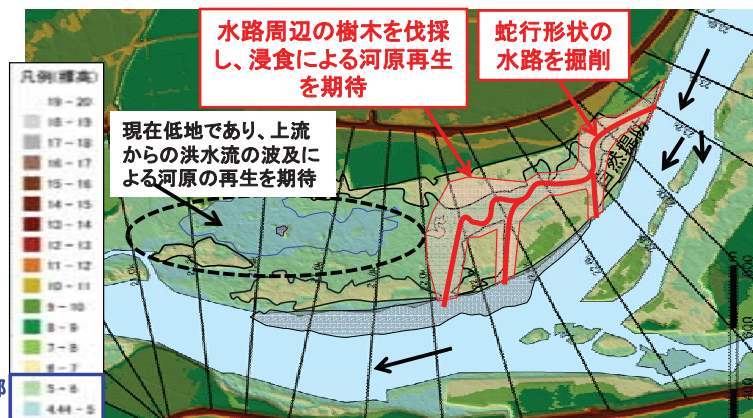
図 4.5-7 水ヶ曾根地区の平面形状（案）
