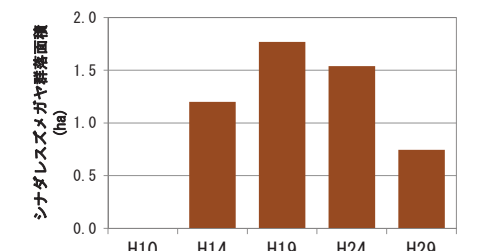
図 3.2-29 右岸河口部「松浜の池(トンボ池)」付近への外来種シナダレスズメガヤの侵入
