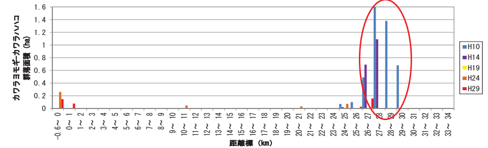
図 3.2-4 カワラヨモギ・カワラハハコ群落面積
