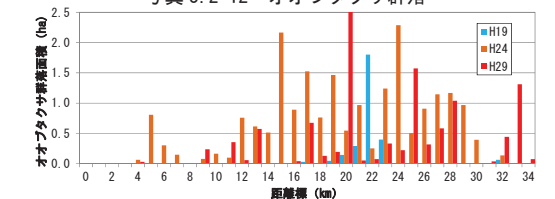
図 3.2-28 H23 出水前後でのオオバクサ群落面積の分布
