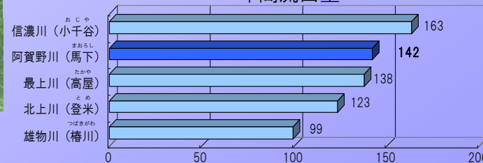
年間流出量
