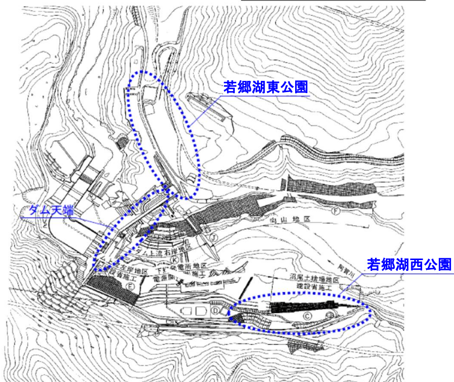
大川ダム点検対象区域図
