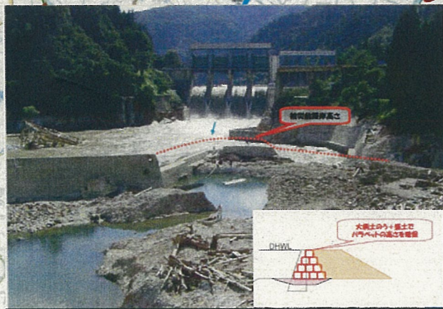
只見川③④ 本名ダム下流 応急工事箇所
