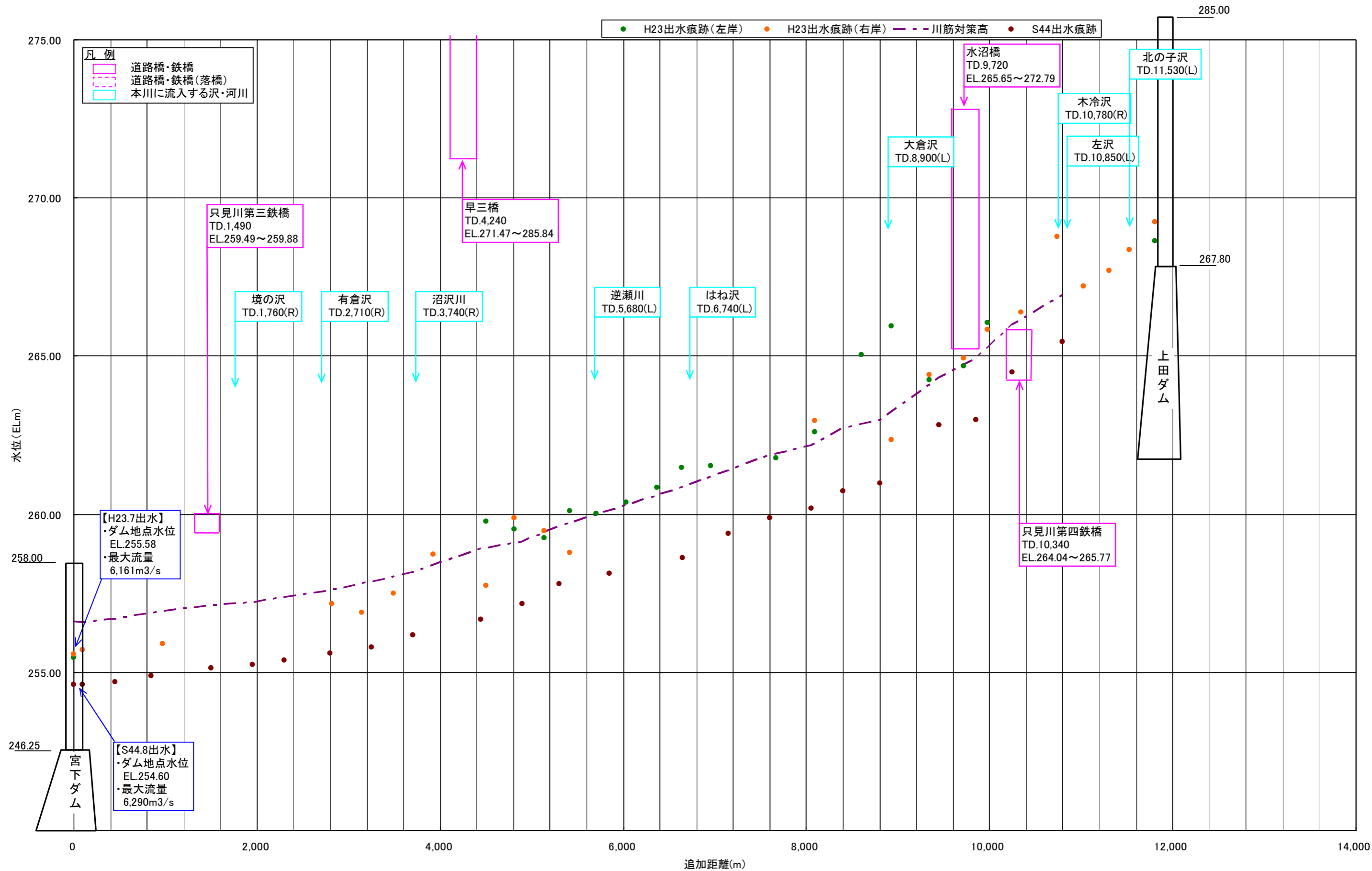
平成23年7月新潟・福島豪雨 宮下ダム調整池洪水痕跡図(速報値)
