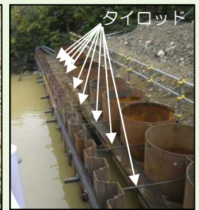
タイロッド設置完了
