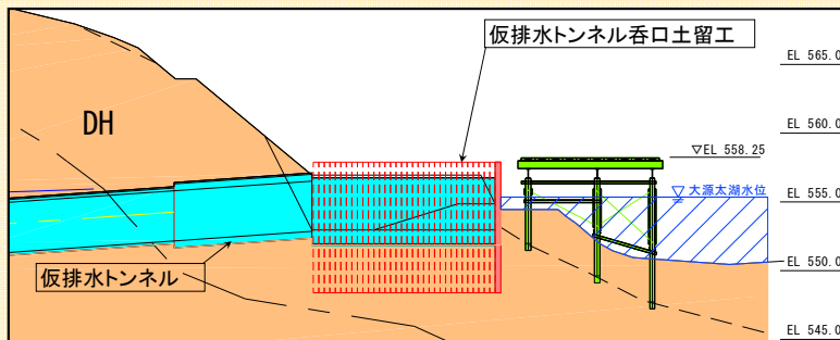
図 仮排水トンネル呑口土留工断面図
