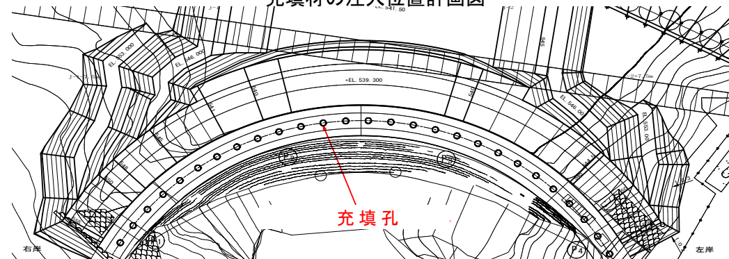
充填材の注入位置計画図
