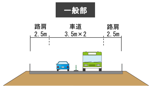
標準横断面図(暫定2車線)
