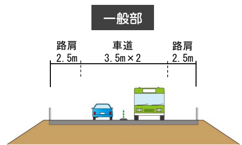
標準横断面図（暫定2車線）
