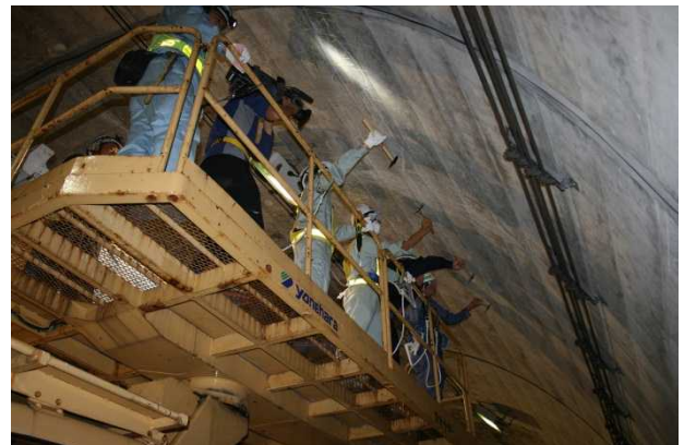
(テストハンマーによる打音点検状況)
