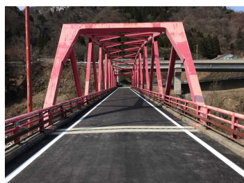
〈トラス部 腐食状況〉
