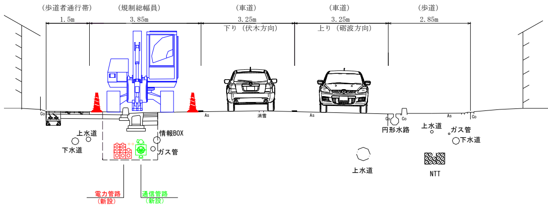
規制断面(車道幅員3.25m)
