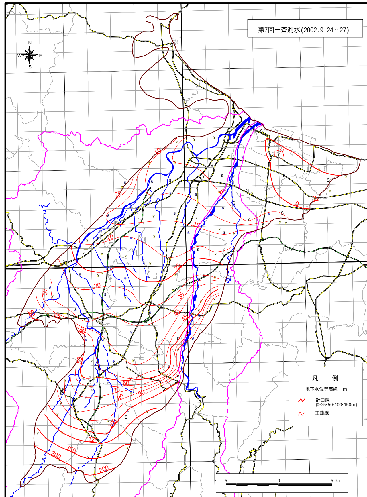
地下水位等高線図 (2002年9月)
