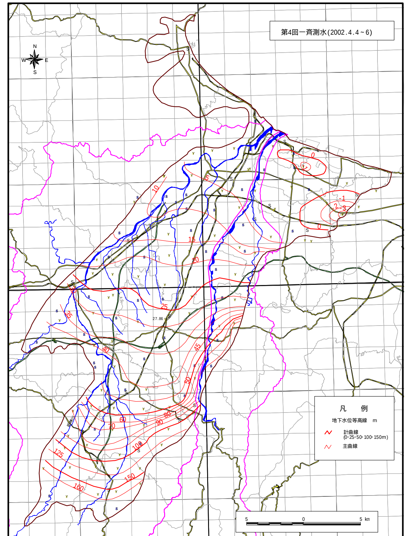
地下水位等高線図 (2002年4月)
