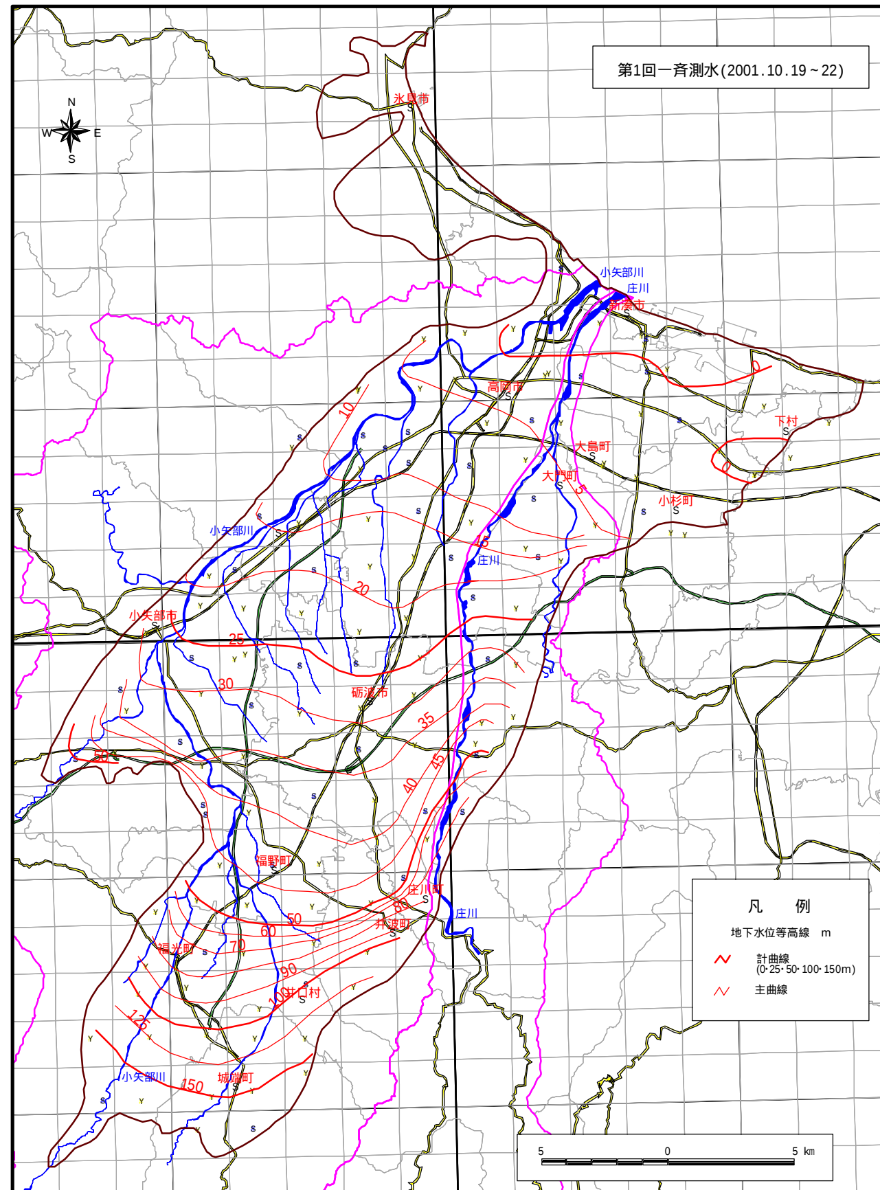
地下水位等高線図 (2001年10月)
