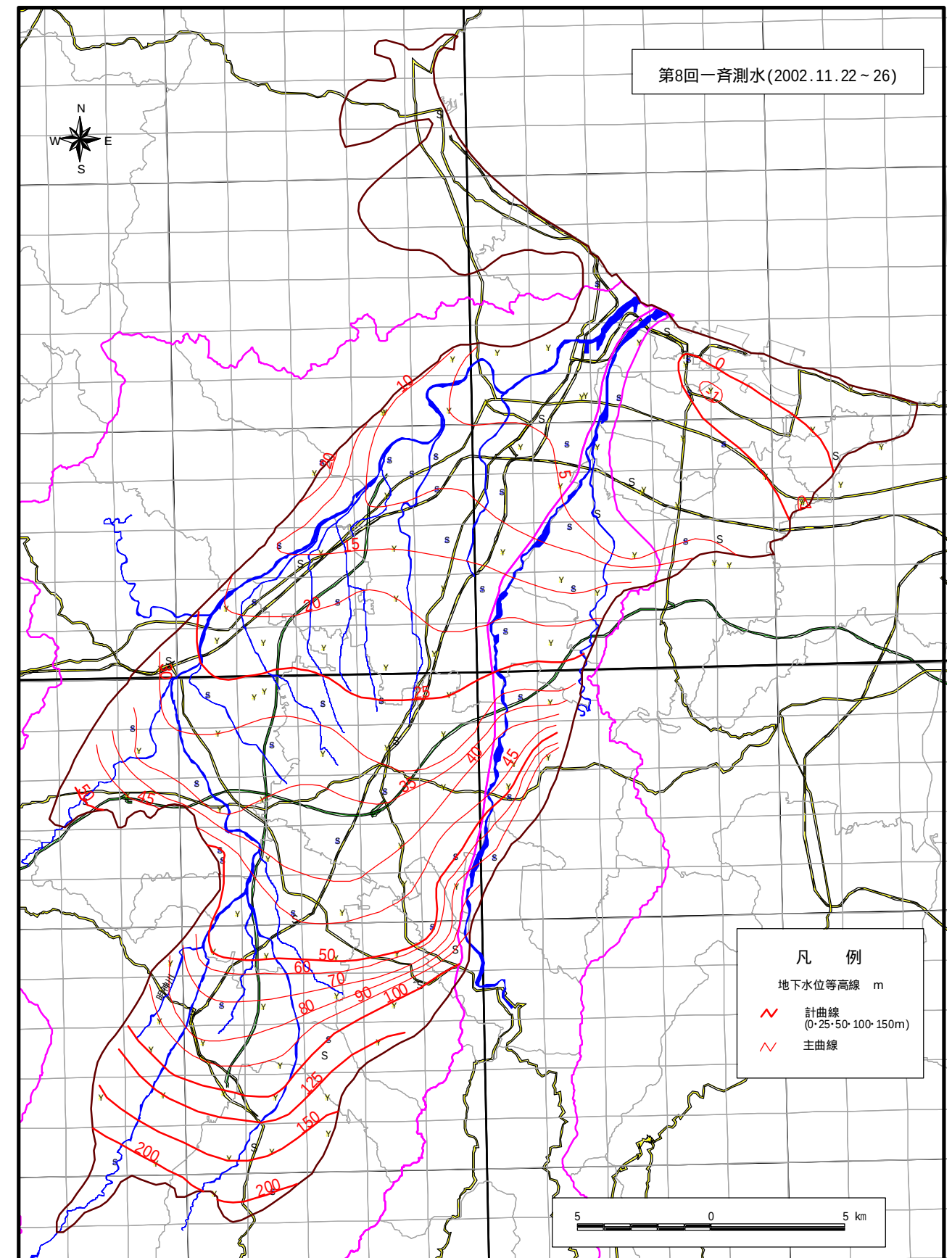
地下水位等高線図 (2002年11月)
