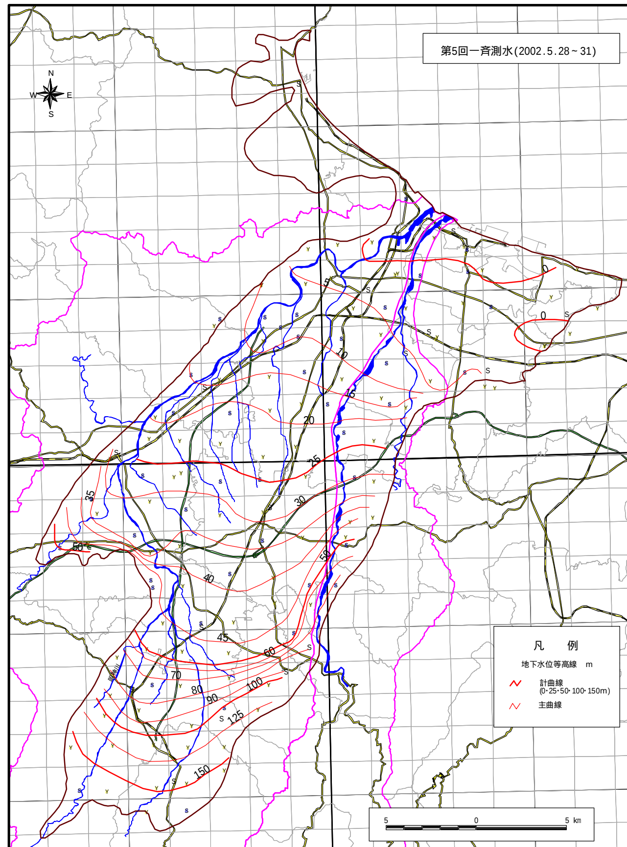
地下水位等高線図(2002年5月)
