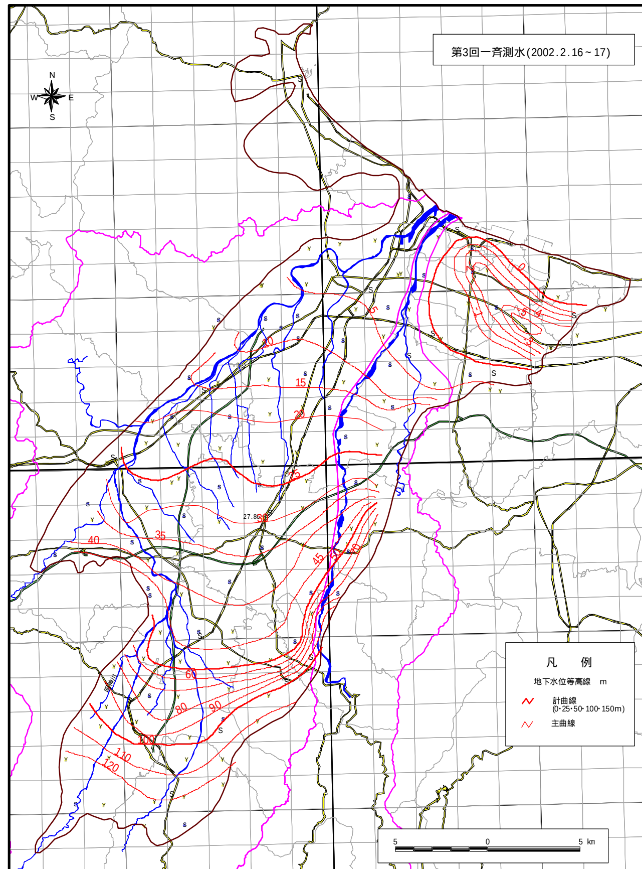
地下水位等高線図 (2002年2月)
