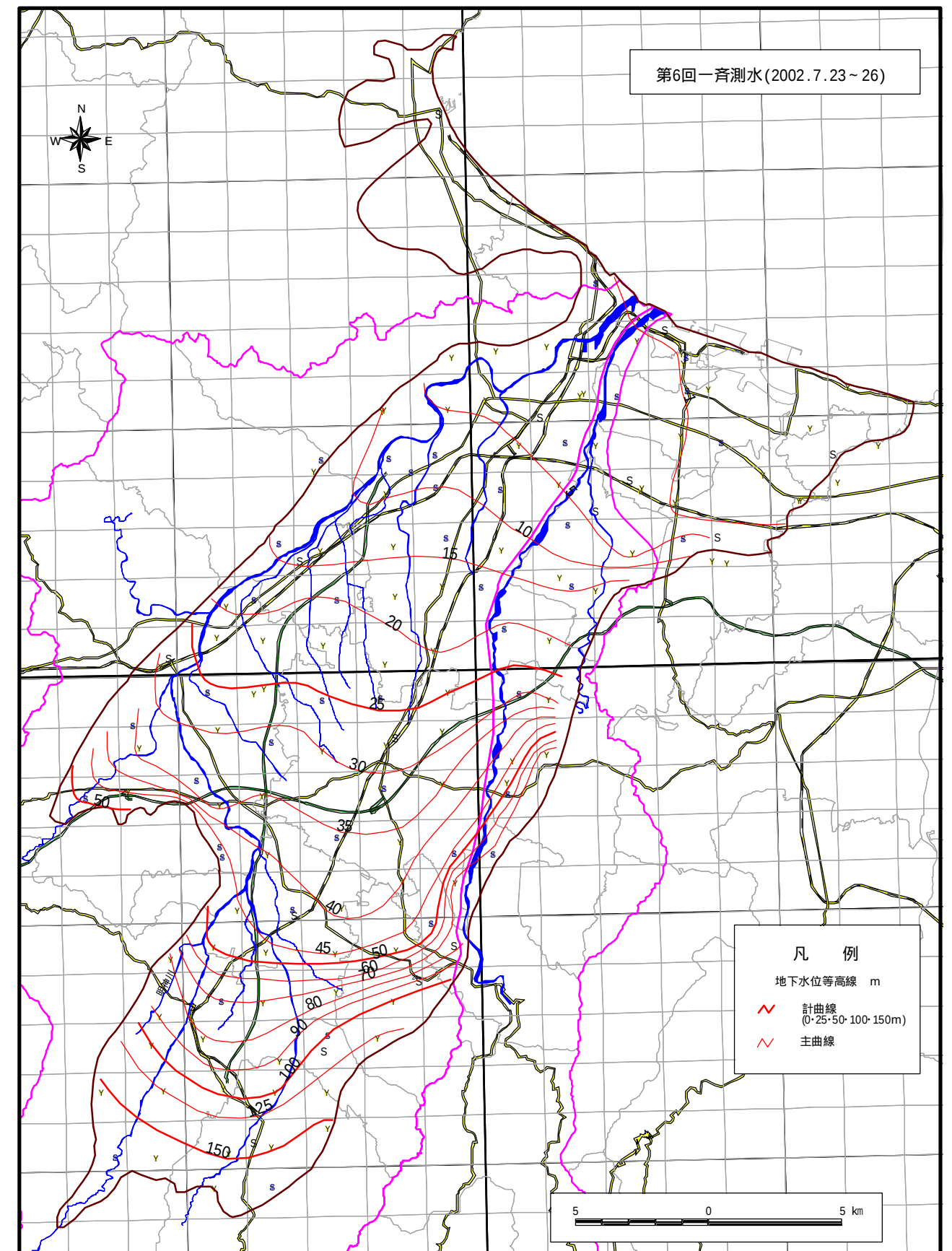
地下水位等高線図(2002年7月)
