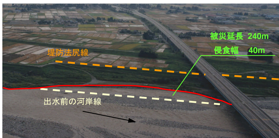
図 3.9 平成10年8月7日洪水による被災状況
