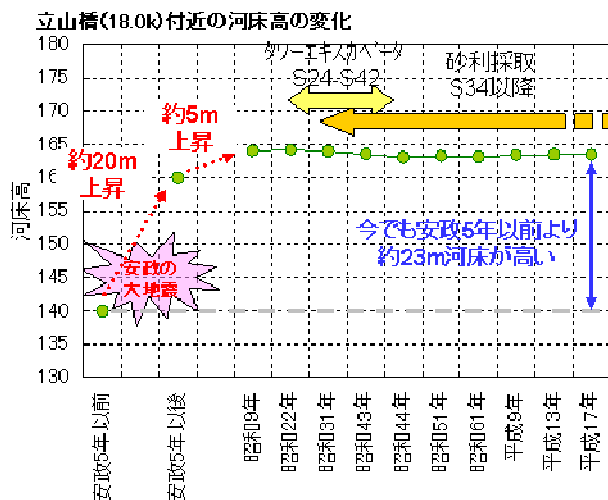
図 3.6 安政の大地震による河床高の変化
