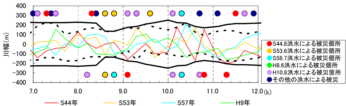
図 3.18 河床の変化と既往の被災箇所
