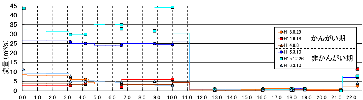
図 3.44 同時流量観測結果
