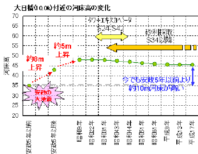
図 3.6 安政の大地震による河床高の変化
