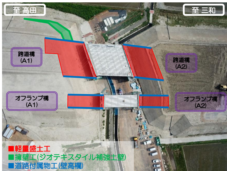
【施工範囲図】
