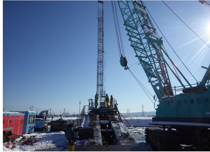
施工状況(戸野目川上流側道橋 下部工)
