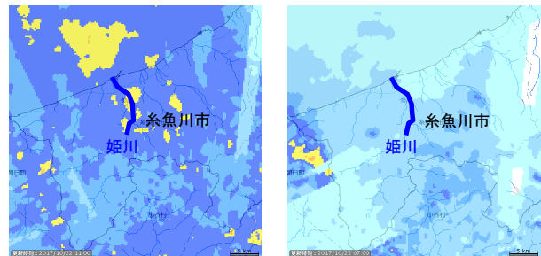
姫川レーダ雨量図 (10月22日 11:00) 姫川レーダ雨量図 (10月23日 7:00) ※レーダ雨量画像は、XRAINホームページより
