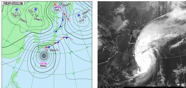
※地上天気図、ひまわり8号画像は、気象庁ホームページより
