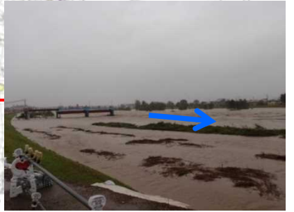
関川R7.6k 10月23日 AM 9:00
