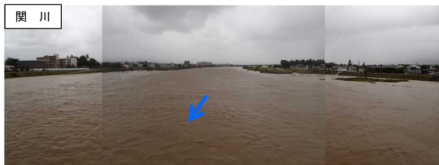
関川 稲田橋上流(10月23日 11:00頃の状況)
