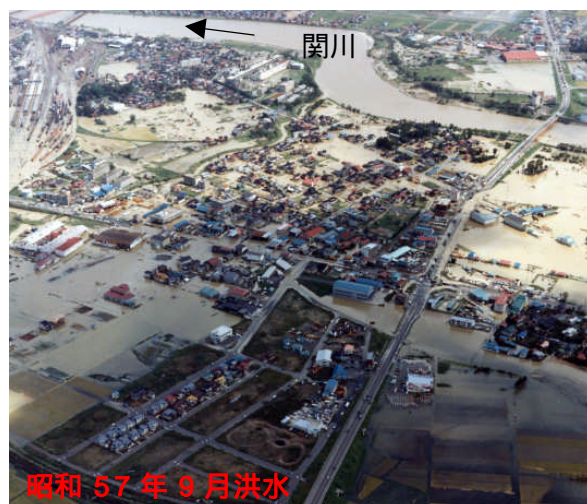
上空より関川大橋を望む
