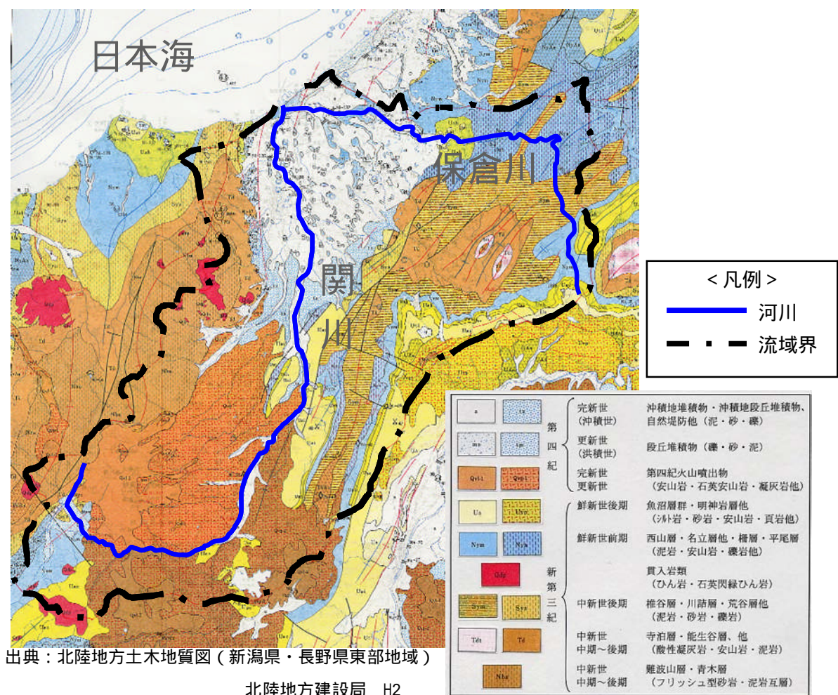
図 2-2 関川流域地質図
