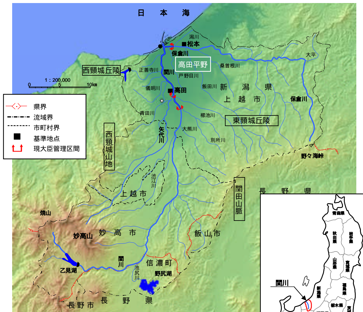
図 2-1 関川水系流域図
