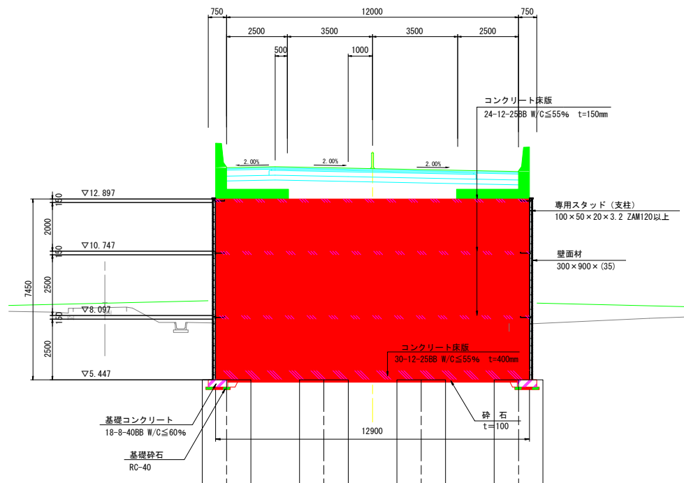
【標準断面図】
