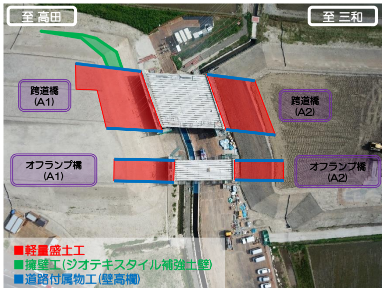
【施工範囲図】
