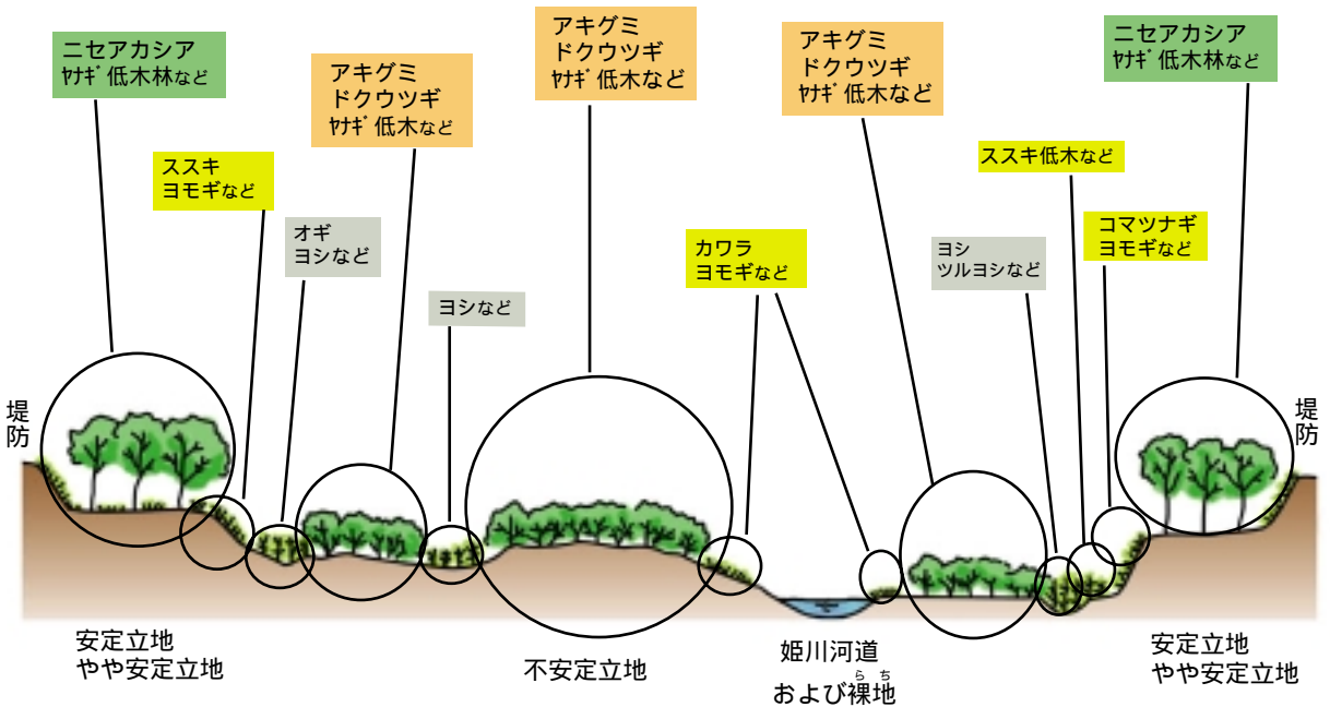
図 - 2 姫川の植物群落の横断模式図
