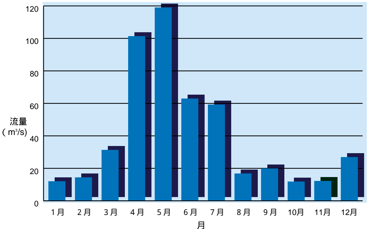
S62～H8年 姫川月別平均流量 ( 中山橋付近 )
