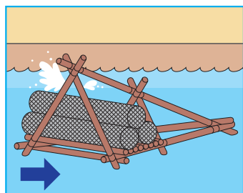
かわくらこう 川倉工 堤防にあたる水の流れを緩やかにして、洗掘が広がるのを防ぐ工法
