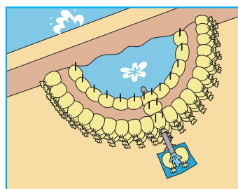
月の輪工 堤防の裏側の水が噴き出した部分に、土のうを積み重ねて水を貯めることで水圧を弱め、吹出し口が広がるのを防ぐ工法
