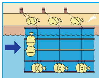
シート張り工 防水シートなどで堤防斜面を覆い堤防の崩れや河川の水のしみ込みを防ぐ工法
