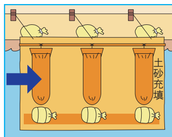
T型マット工 水防マットを使用して堤防斜面を覆い堤防の崩れや河川の水のしみ込みを防ぐ工法
