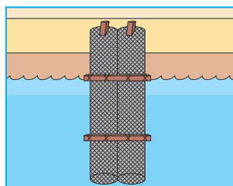
たてじゃかごこう 立蛇籠工 川側堤防斜面に蛇かごを立てて被覆する工法。過去に洗掘、欠損した箇所に災害が再発するのを防ぐ
