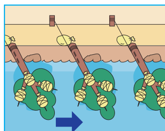
木流し工 木に重しをつけて川の中に流し、堤防に当たる流れの勢いを弱める工法
