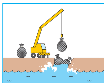
袋詰め玉石工 合成繊維を使用した網状の袋材に玉石等を袋詰めし、クレーンで吊り、洗掘箇所を設置し、堤防を補強する工法
