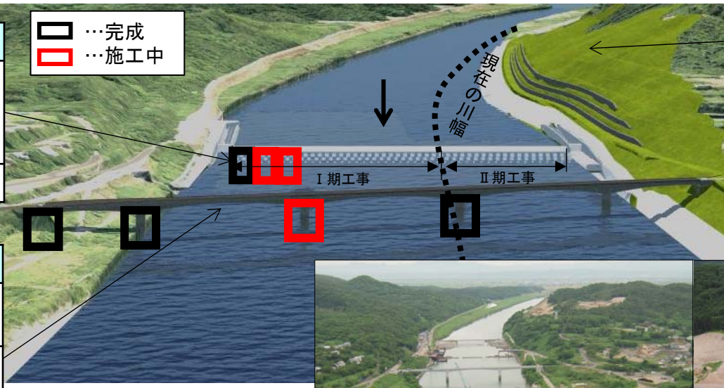
大河津分水路改修完成予想図 (河口より上流を望む)
