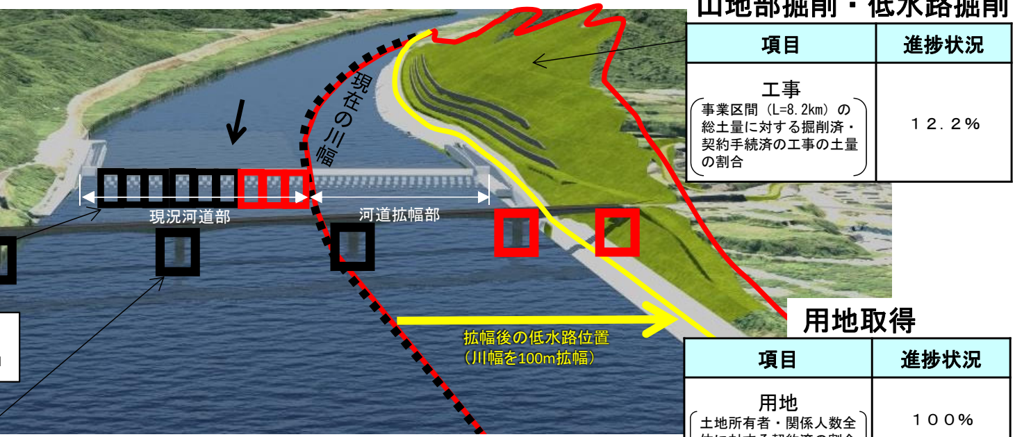
大河津分水路改修完成予想図 (河口より上流を望む)
