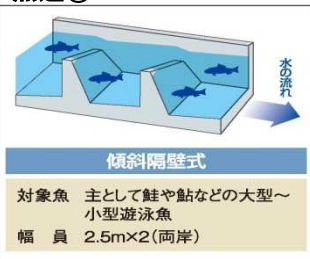
可動堰に設置されている魚道の種類
