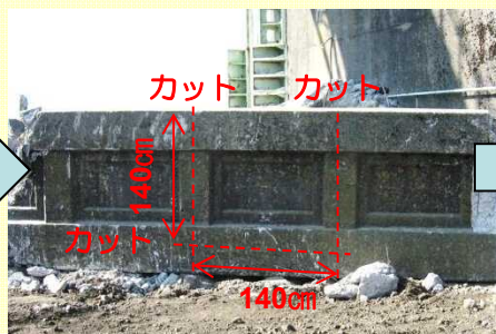
撤去した高欄を加工
