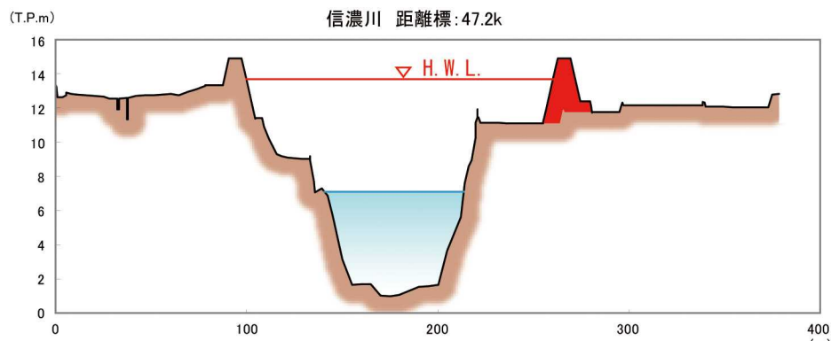
図 42 堤防整備断面のイメージ図(下流部)
