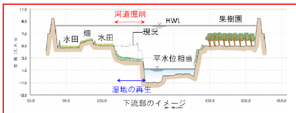
図 45 河道掘削断面のイメージ図（下流部）
