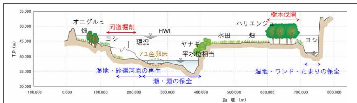
図 44 河道掘削断面のイメージ図(中流部)
