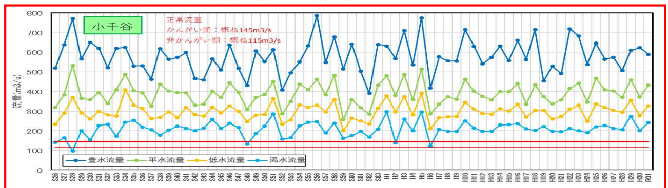
図 25 河川流況 (小千谷地点)
