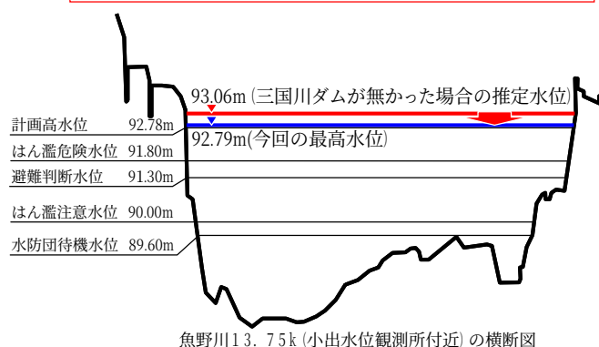
図 16 平成 23 年 7 月洪水時における三国川ダムの洪水調節の様子
