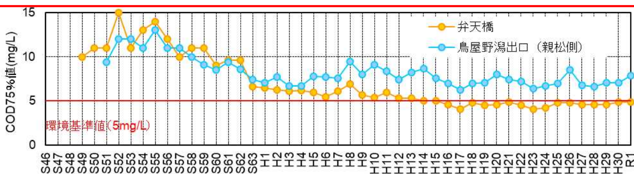
図 28 鳥屋野潟の COD75%値の推移
