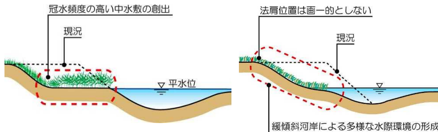
図 47 中流部における環境に配慮した掘削形状イメージ図
