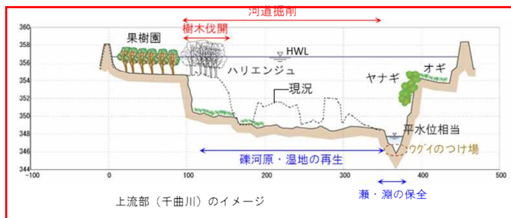
図 43 河道掘削断面のイメージ図(上流部)
