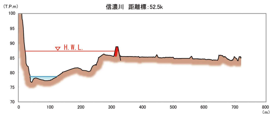
図 41 堤防整備断面のイメージ図(中流部)
