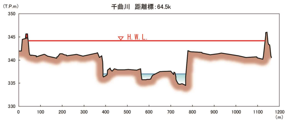
図 40 堤防整備断面のイメージ図(上流部)
