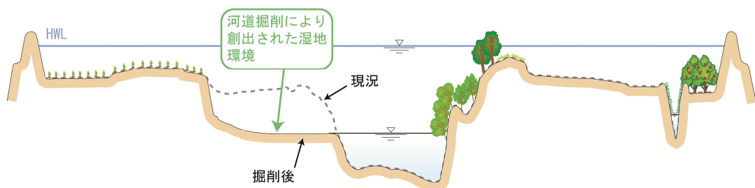
図 48 下流部における環境に配慮した掘削形状イメージ
