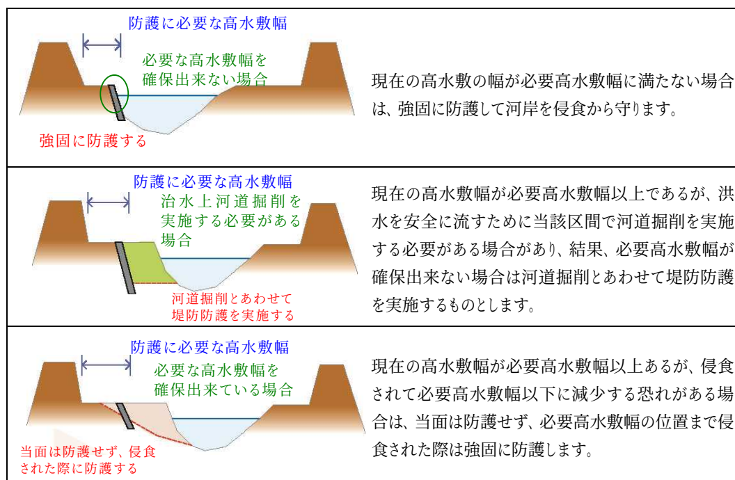
図 51 高水敷幅による堤防防護の考え方
