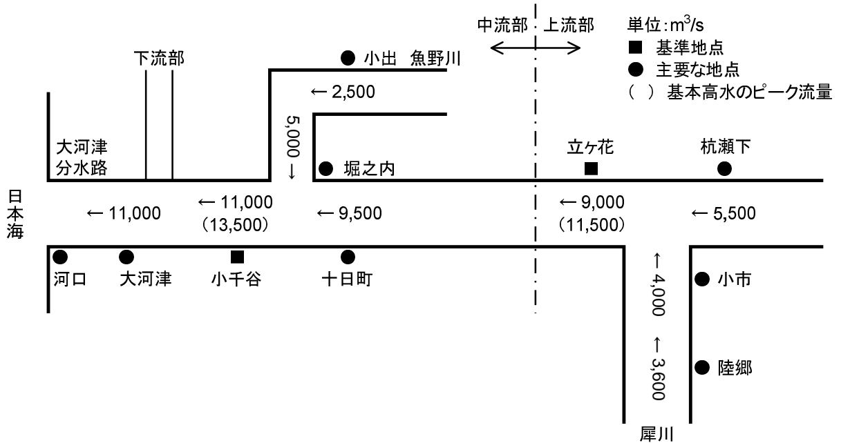
図6 河川整備基本方針における上流部・中流部計画高水流量図 (単位:m 3 /s)
