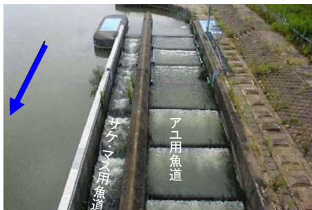
蒲原大堰に設置された魚道
