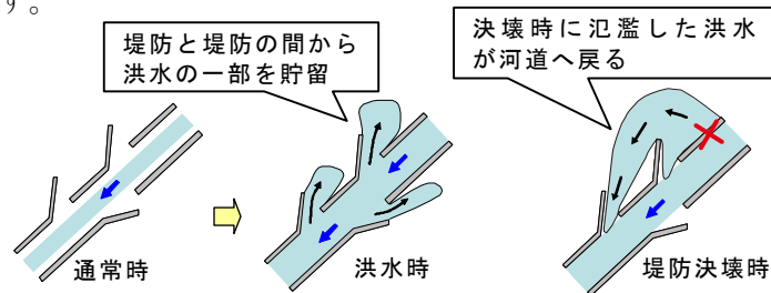
図 16 霞堤の効果
