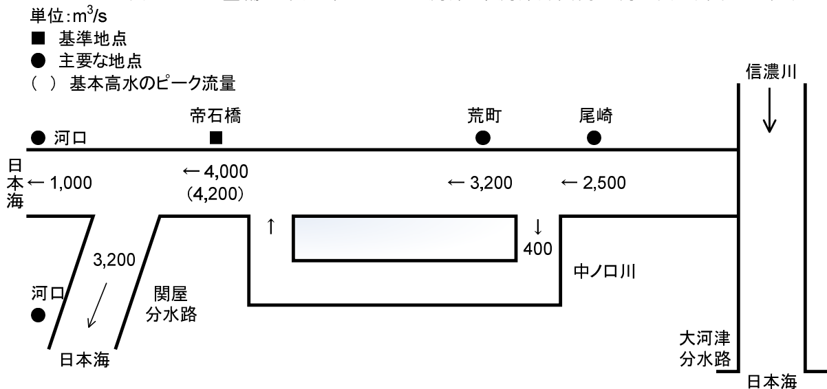
図7 河川整備基本方針における下流部計画高水流量図 (単位:m 3 /s)
