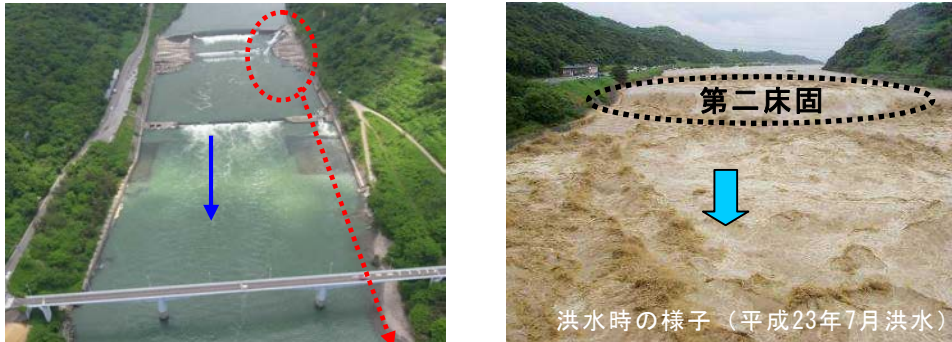
第二床固のひび割れ発生状況 (平成21年調査)
