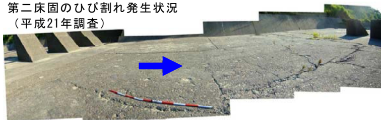
写真 17 大河津分水路 第二床固の老朽化状況
