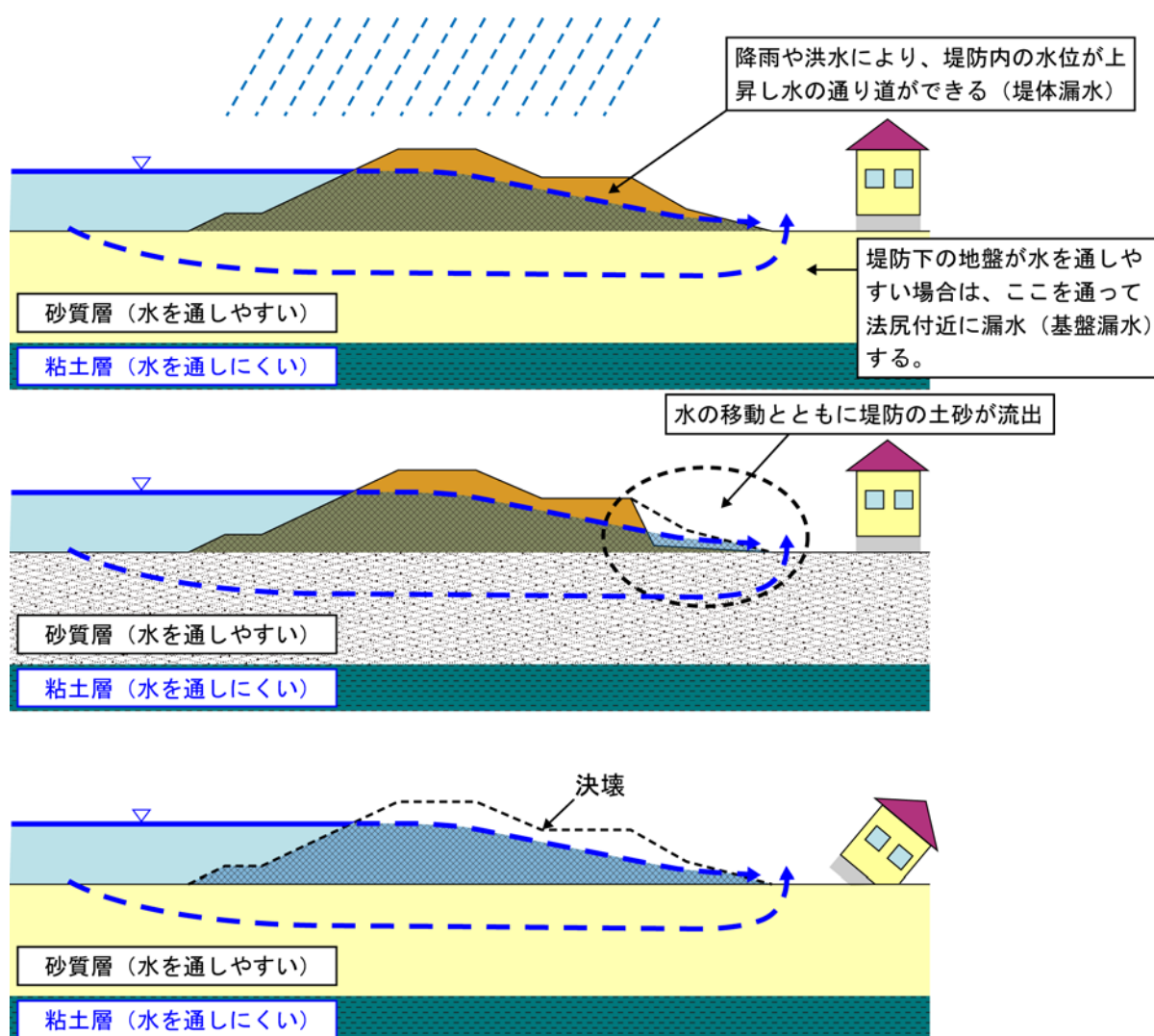
図 13 浸透による堤防の決壊メカニズム
