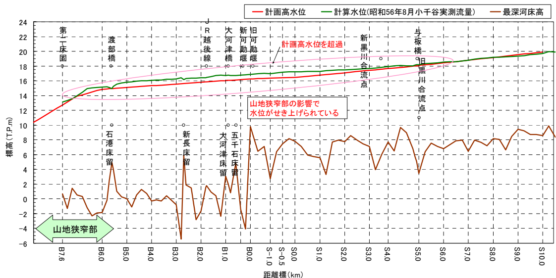
図9 昭和56年8月洪水水位縦断面図(河口～信濃川10.0km)
