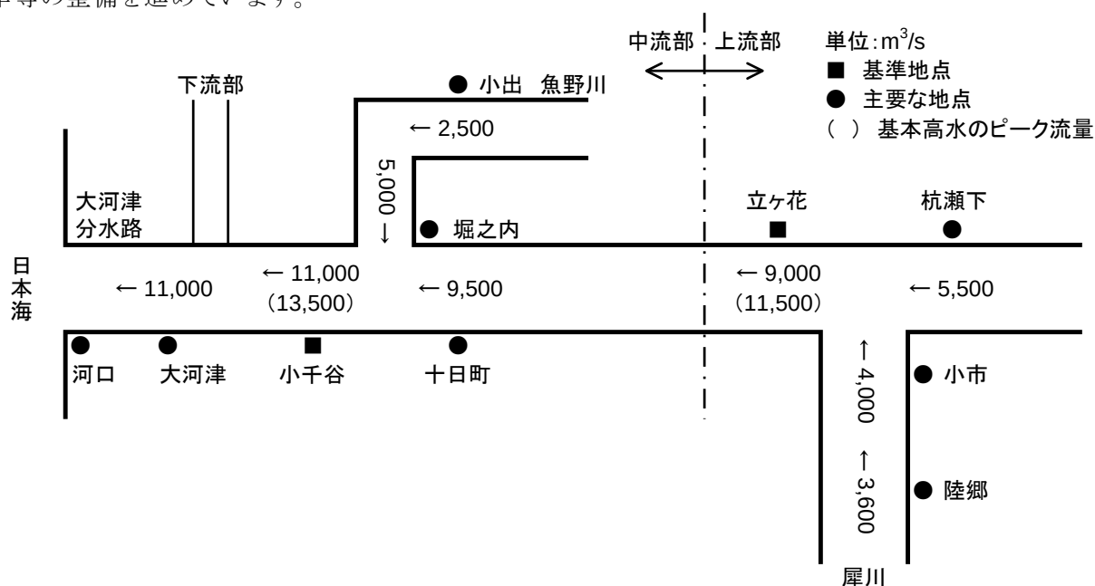
図6 河川整備基本方針における上流部・中流部計画高水流量図 (単位: \text{m}^3/\text{s} )
