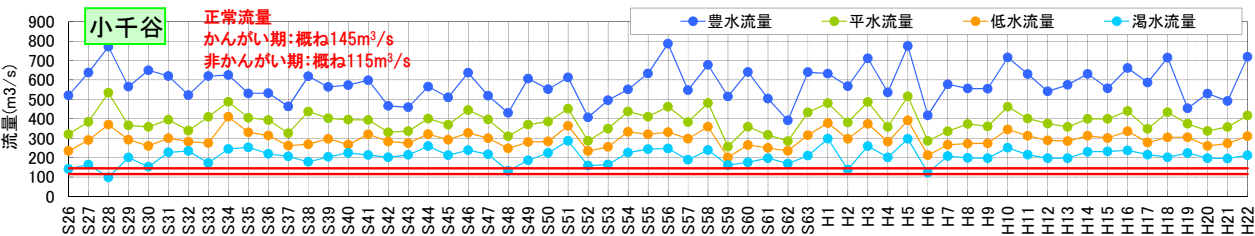
図 17 河川流況(小千谷地点)
