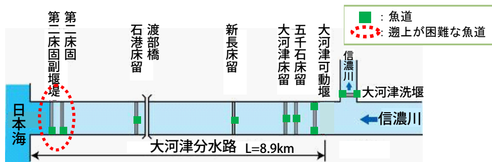
図 33 大河津分水路周辺の魚道設置状況
