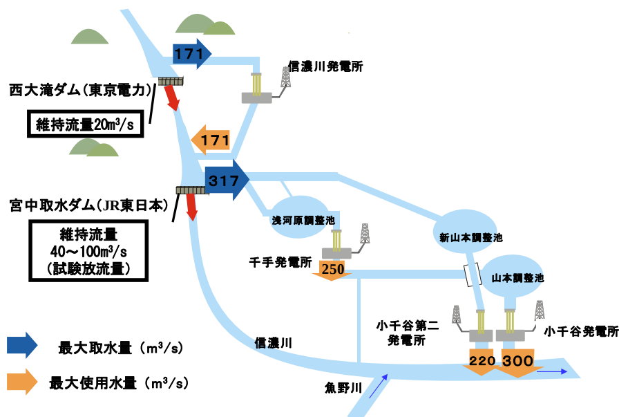
図 16 減水区間の発電取水等模式図
