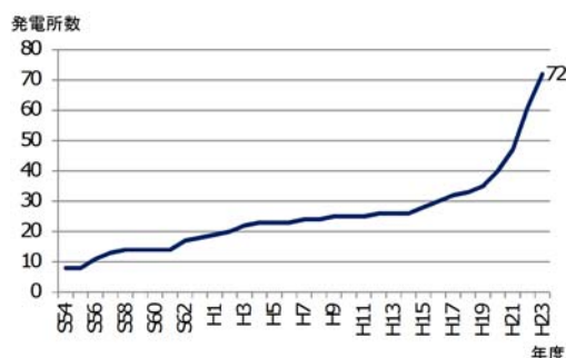
図 15 全国の一級水系における従属発電所(1,000kW 未満)の数(累計)
