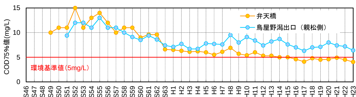
図 19 鳥屋野潟の COD75%値の推移
