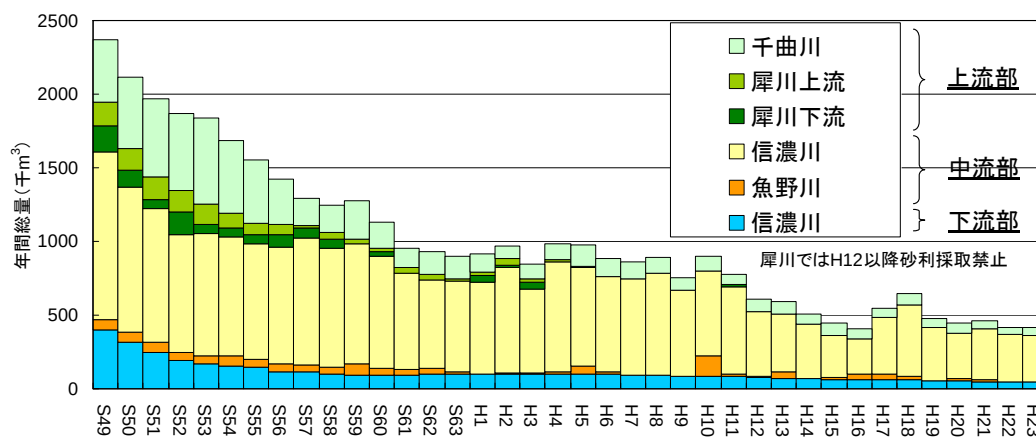
図 25 信濃川水系の砂利採取量の経年変化
