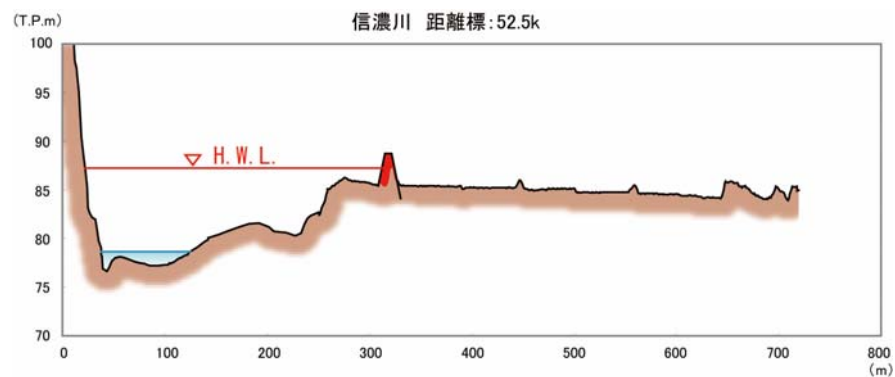
図 29 堤防整備断面のイメージ図(中流部)
