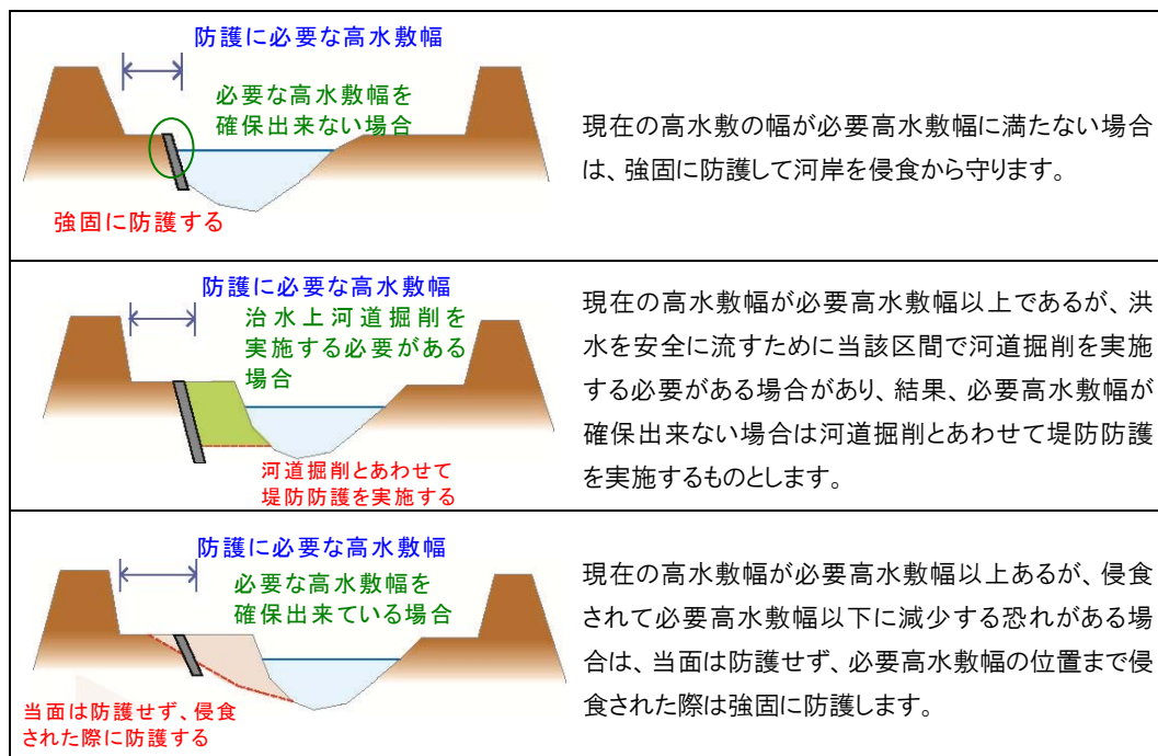
図 35 高水敷幅による堤防防護の考え方
