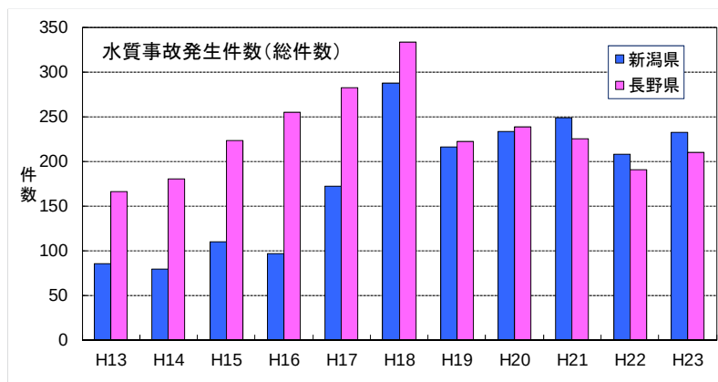
図 20 新潟県と長野県における水質事故の発生状況
