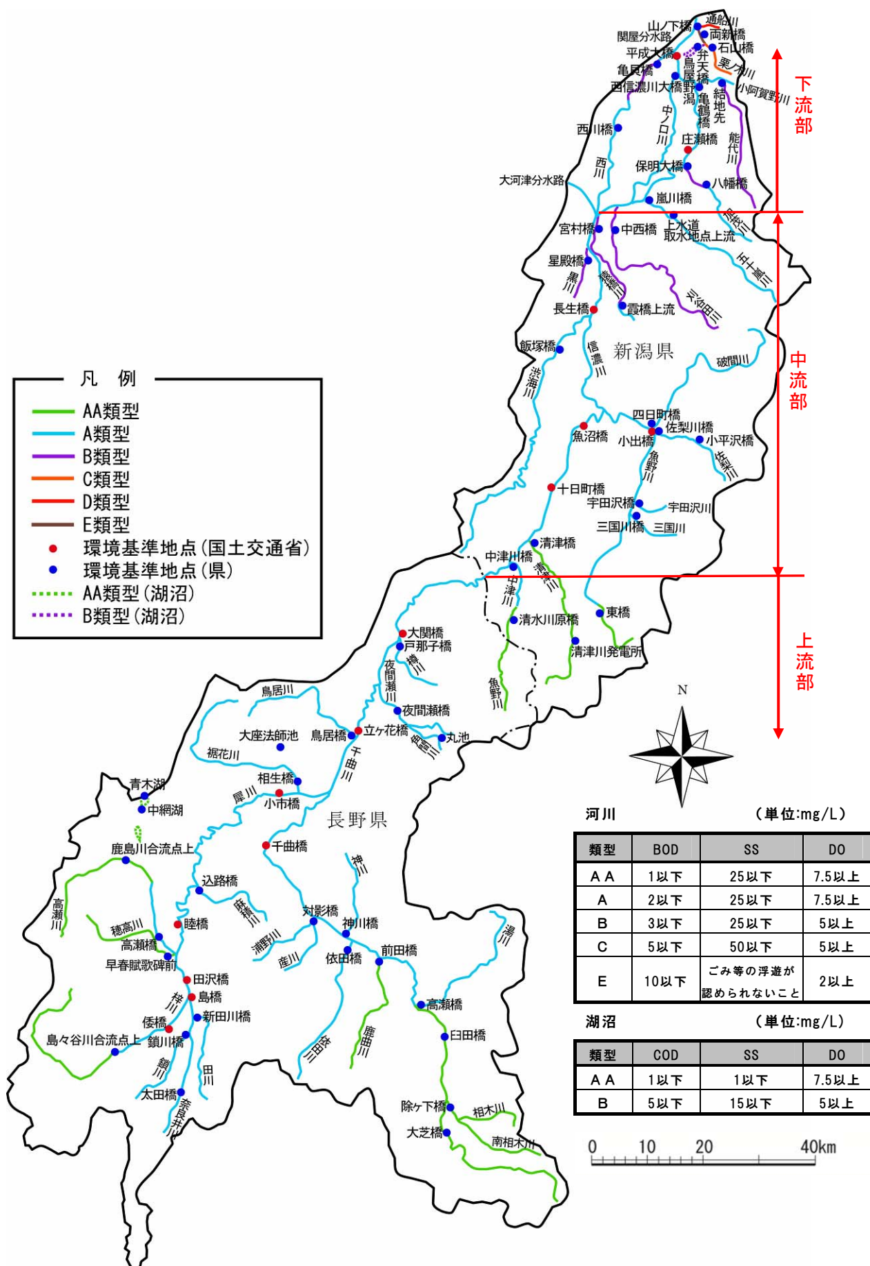
図 21 信濃川水系における河川・湖沼の水質環境基準の類型指定状況
