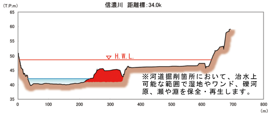
図 30 河道掘削断面のイメージ図(中流部)
