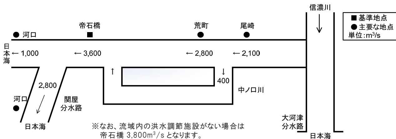
図 27 昭和 58 年 9 月洪水と同規模の洪水(上流部)及び昭和 56 年 8 月洪水と同規模の洪水(中流部)
