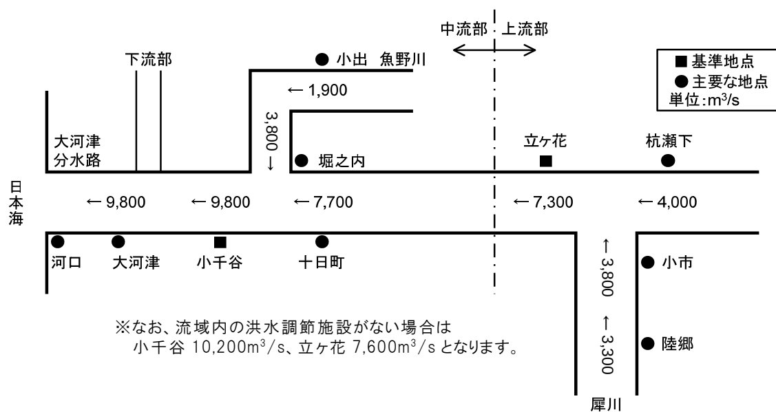
図 27 昭和 58 年 9 月洪水と同規模の洪水(上流部)及び昭和 56 年 8 月洪水と同規模の洪水(中流部)
