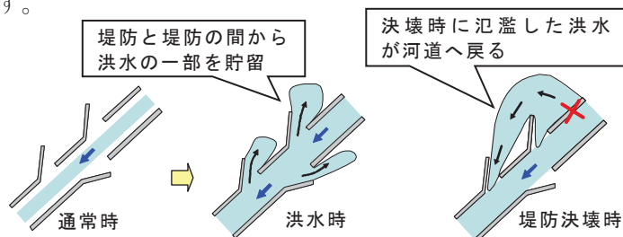
図 16 霞堤の効果
