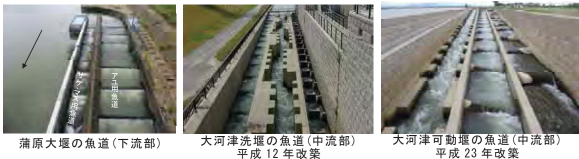
写真 68 魚道の設置事例
