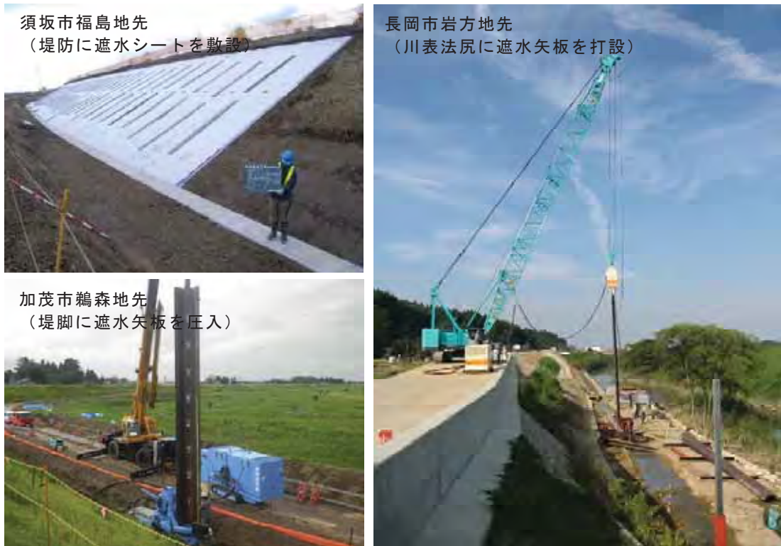
写真 55 浸透対策の実施例
