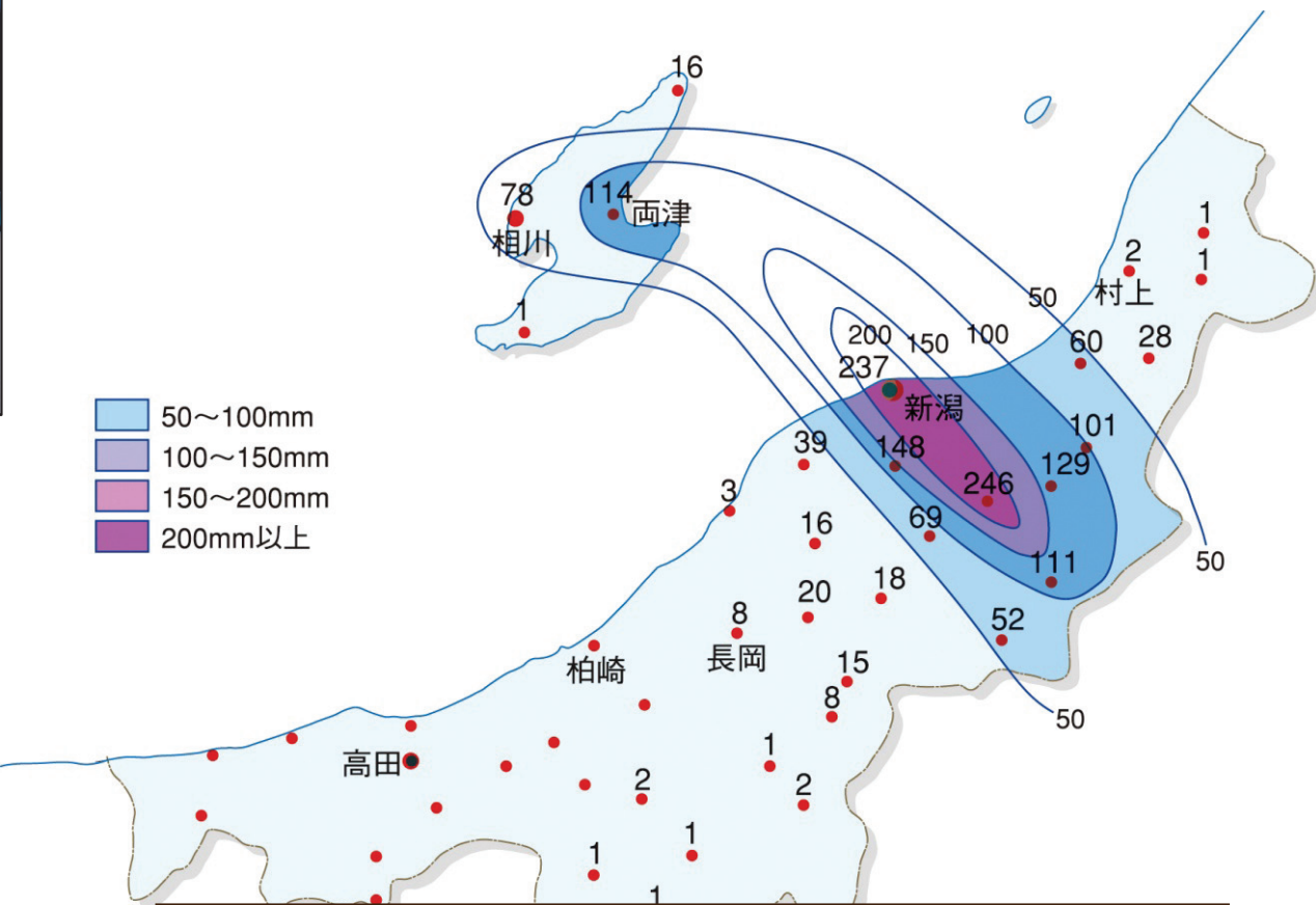
8時間降水量分布図(8月4日0~8時)
