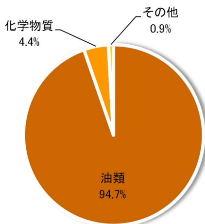
■ 水質事故原因物質（令和元年）
