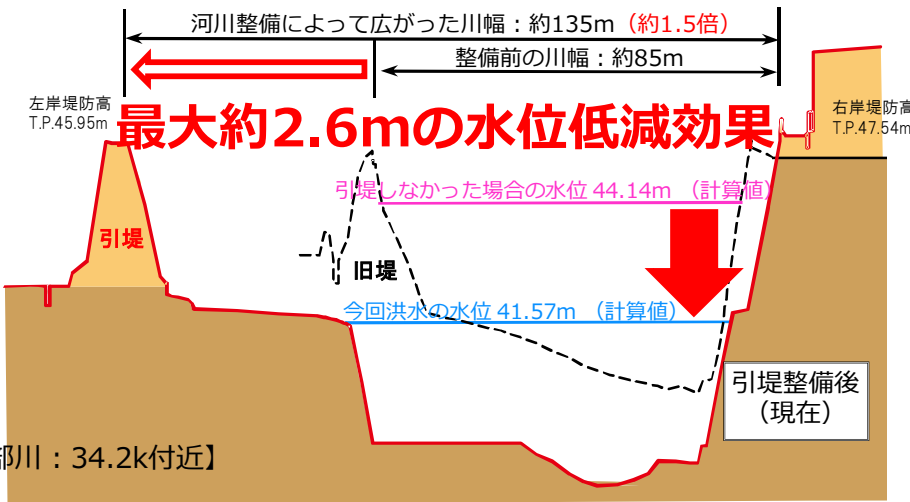
引堤・河道掘削の効果(34.2k付近)
