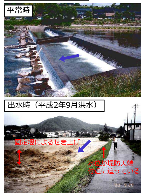
出水状況 井田川左岸14.0k付近（杉原橋観測所）
