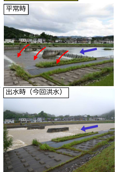
出水状況 井田川左岸14.0k付近（杉原橋観測所）
