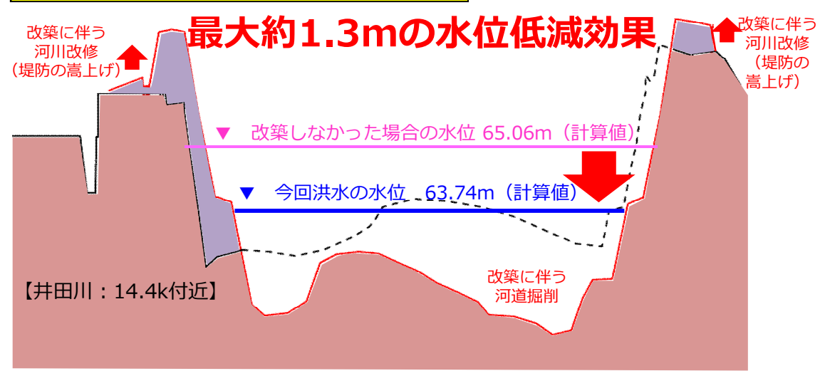
堰改築・河川改修の効果（14.4k付近）
