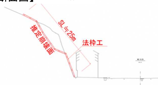
【断面図】 A - A' 断面
