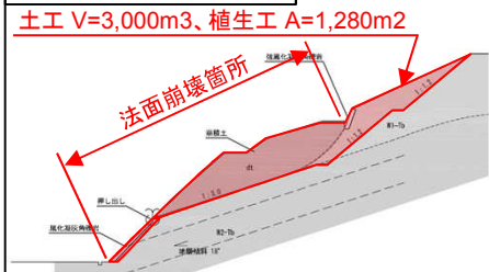
【断面図(A-B断面)】
