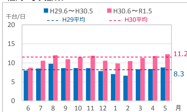
国道8号 宝来
