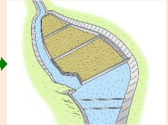
流速が遅くなる遊砂地に、土砂が堆積します。
