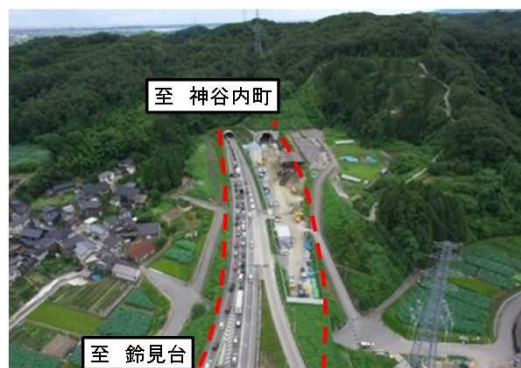
国道159号金沢東部環状道路 舗装工事、トンネル設備工事(石川県)
